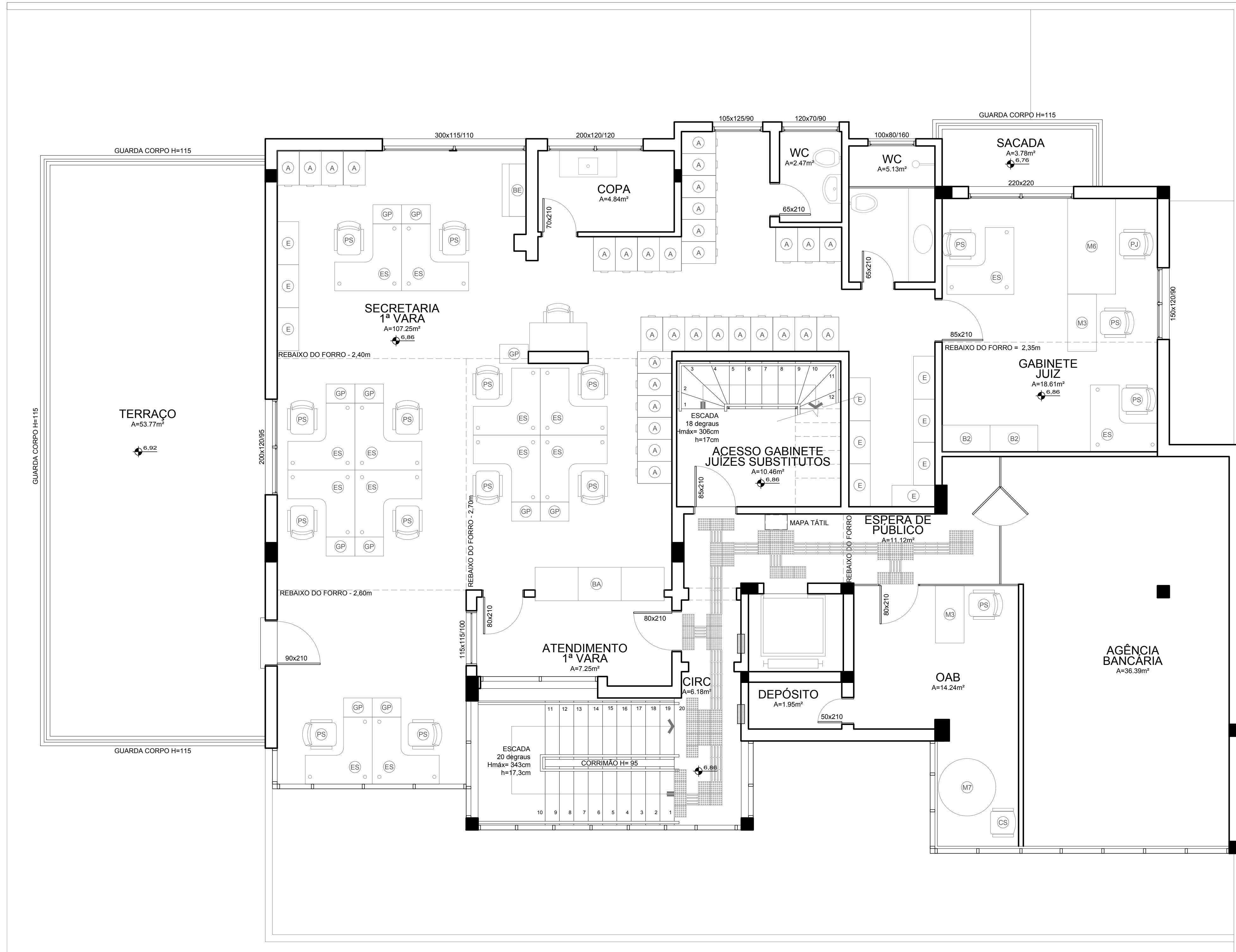
PLANTA BAIXA TERCEIRO PAVIMENTO ESCALA= 1/50
