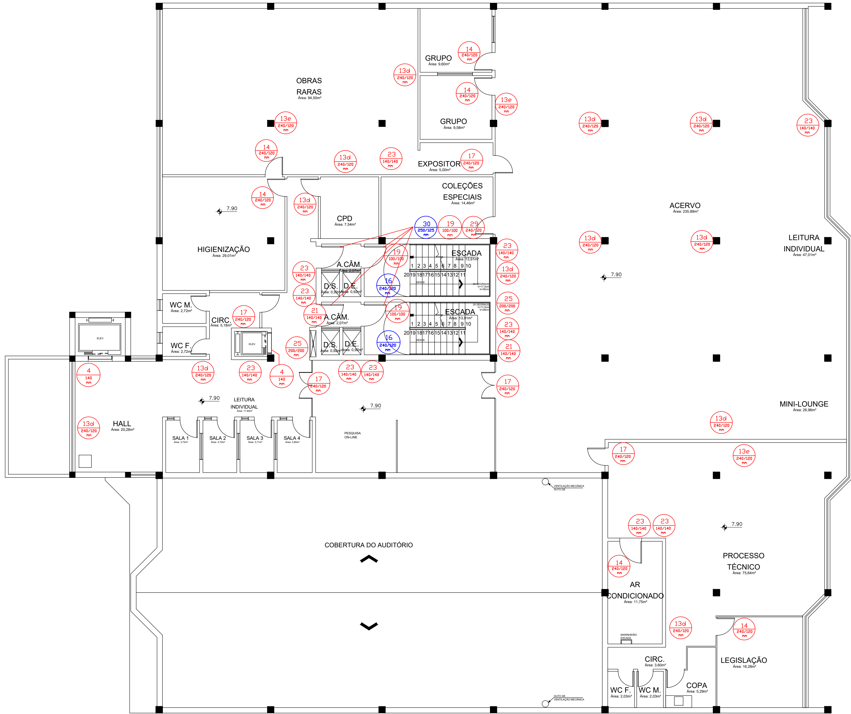
PLANTA BAIXA 2º PAVIMENTO esc.: 1:100
