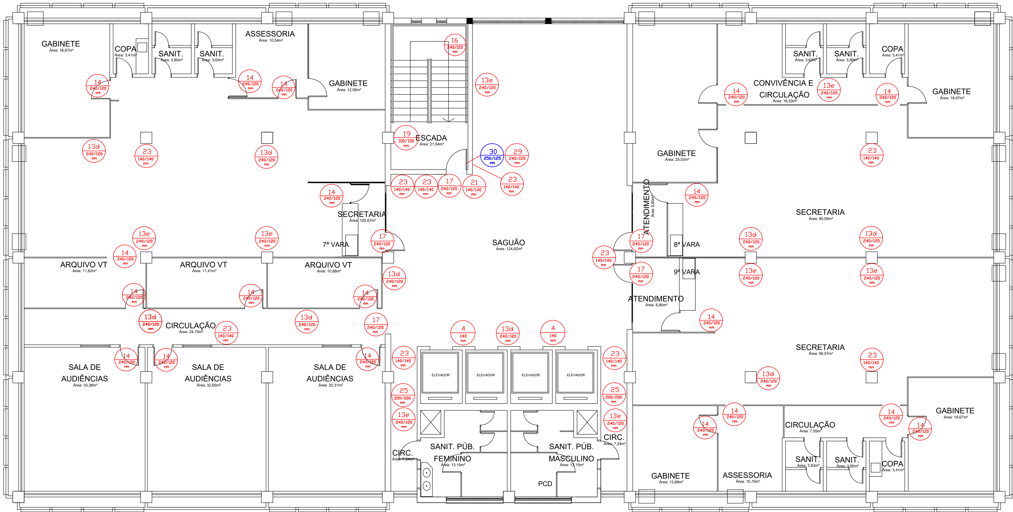
PLANTA BAIXA 4º PAVIMENTO esc.: 1:100
