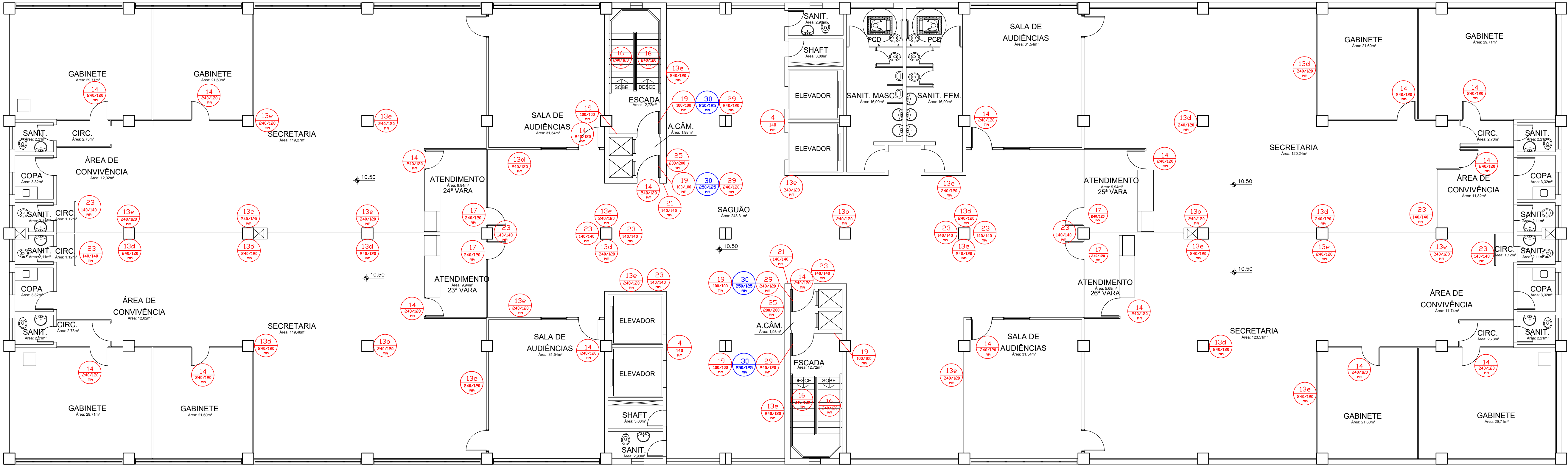
PLANTA BAIXA 3º PAVIMENTO esc.: 1:100
