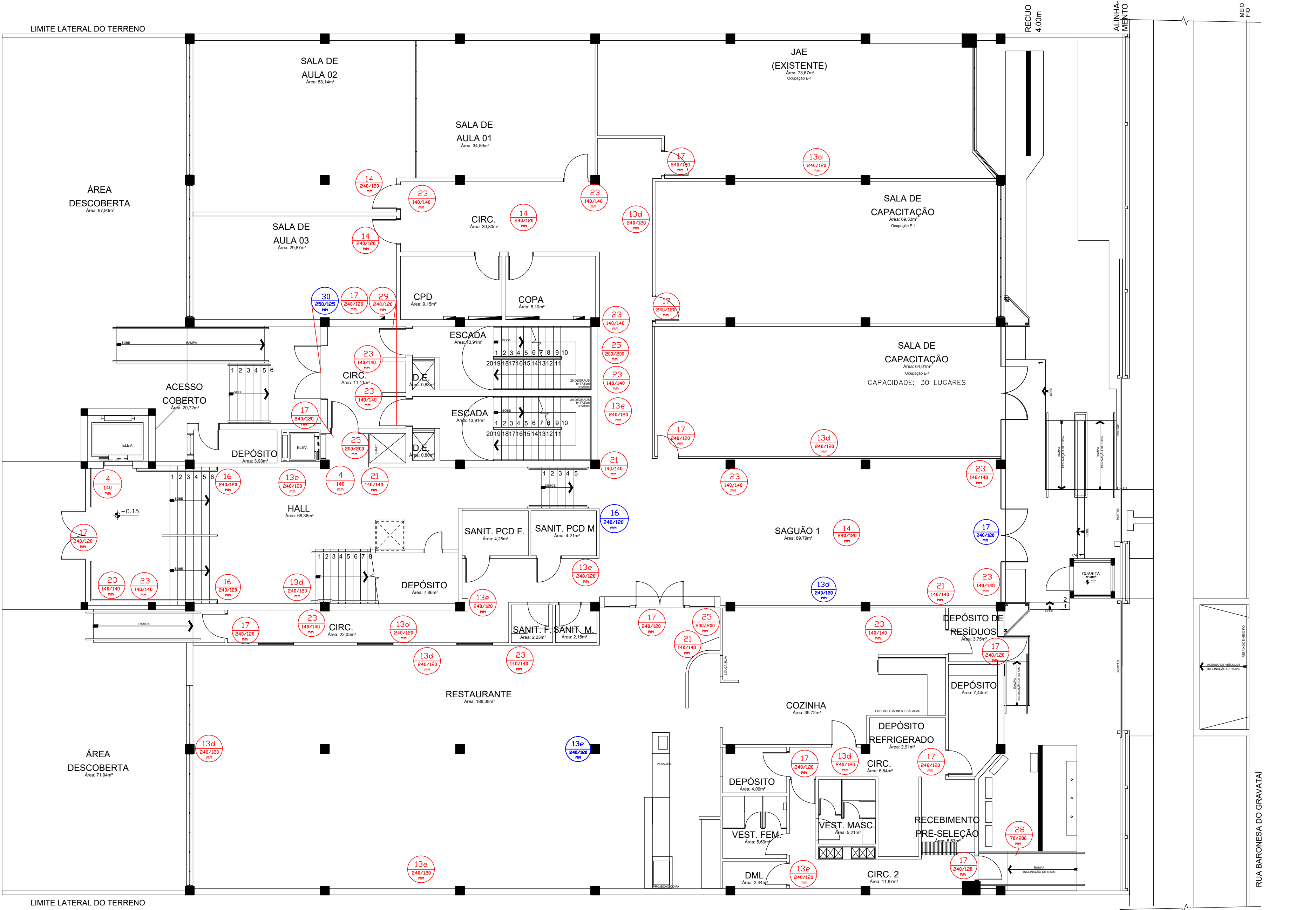
PLANTA BAIXA PAVIMENTO TÉRREO esc.: 1:100
