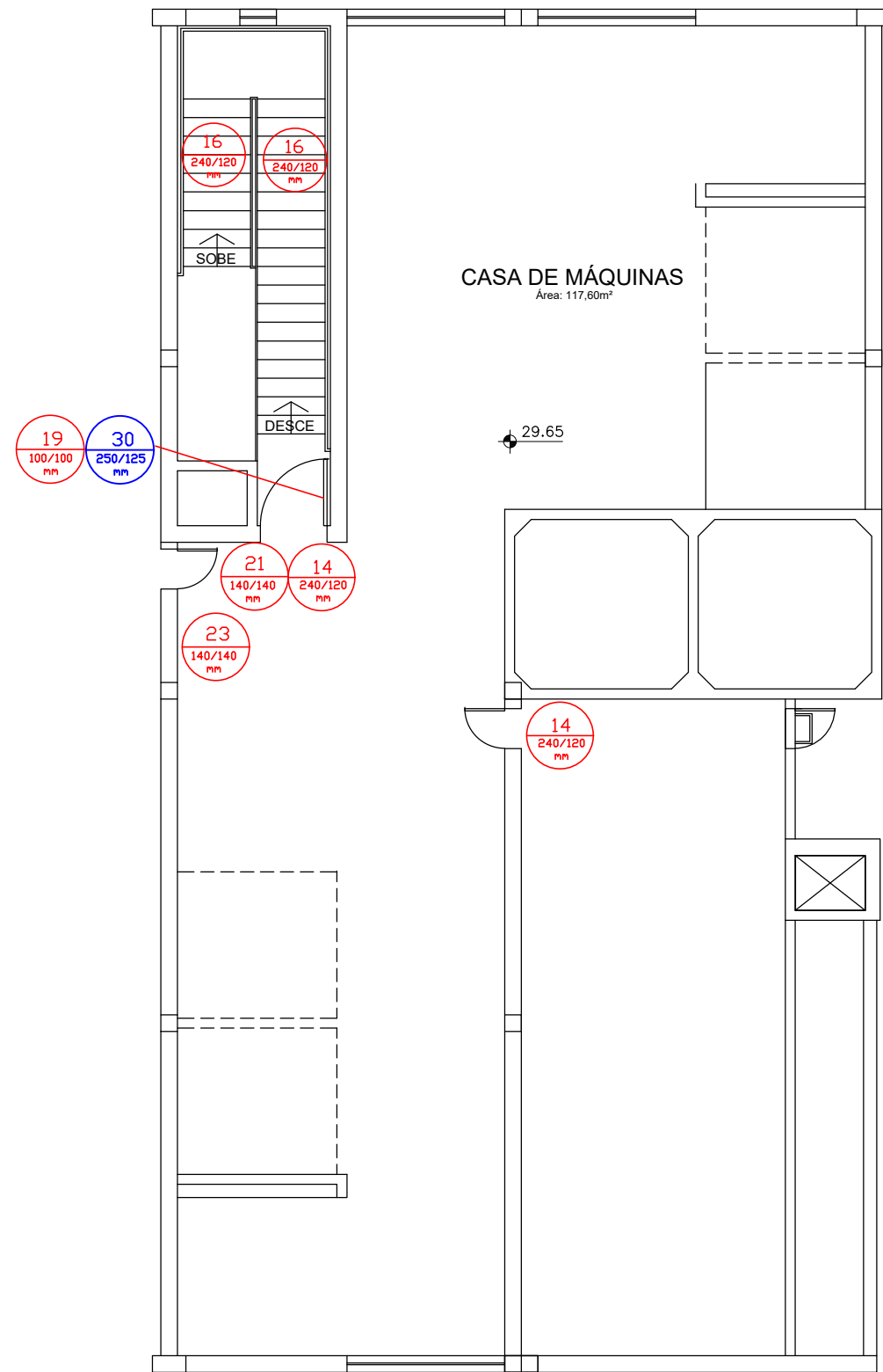
PLANTA BAIXA CASA DE MÁQUINAS CHUVEIRO AUTOMÁTICO esc.: 1:100
