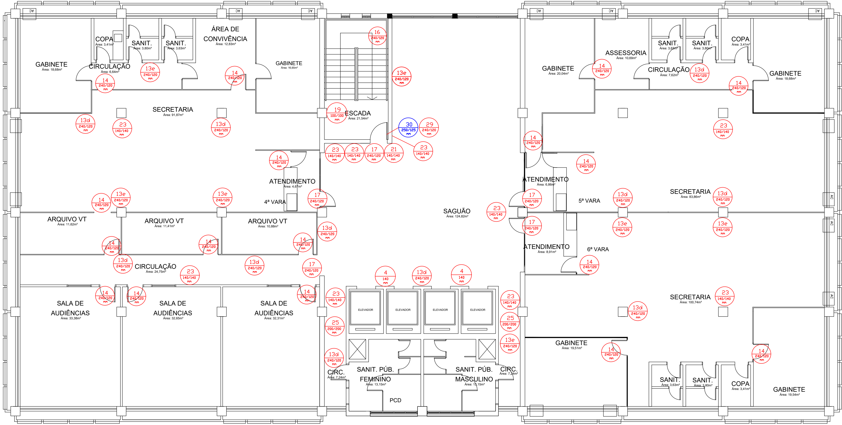
PLANTA BAIXA 3º PAVIMENTO esc.: 1:100
