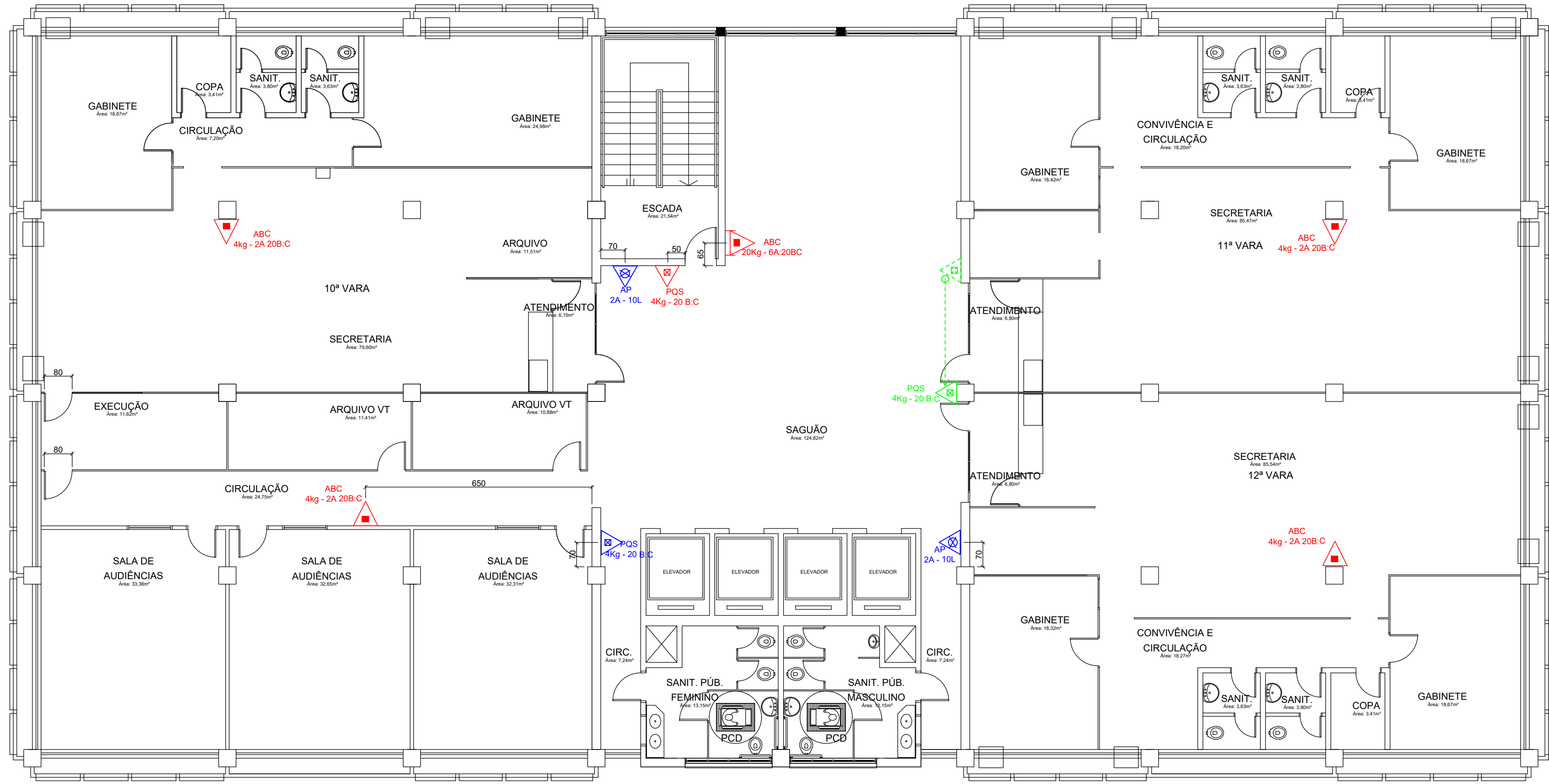
PLANTA BAIXA 5º PAVIMENTO esc.: 1:100
