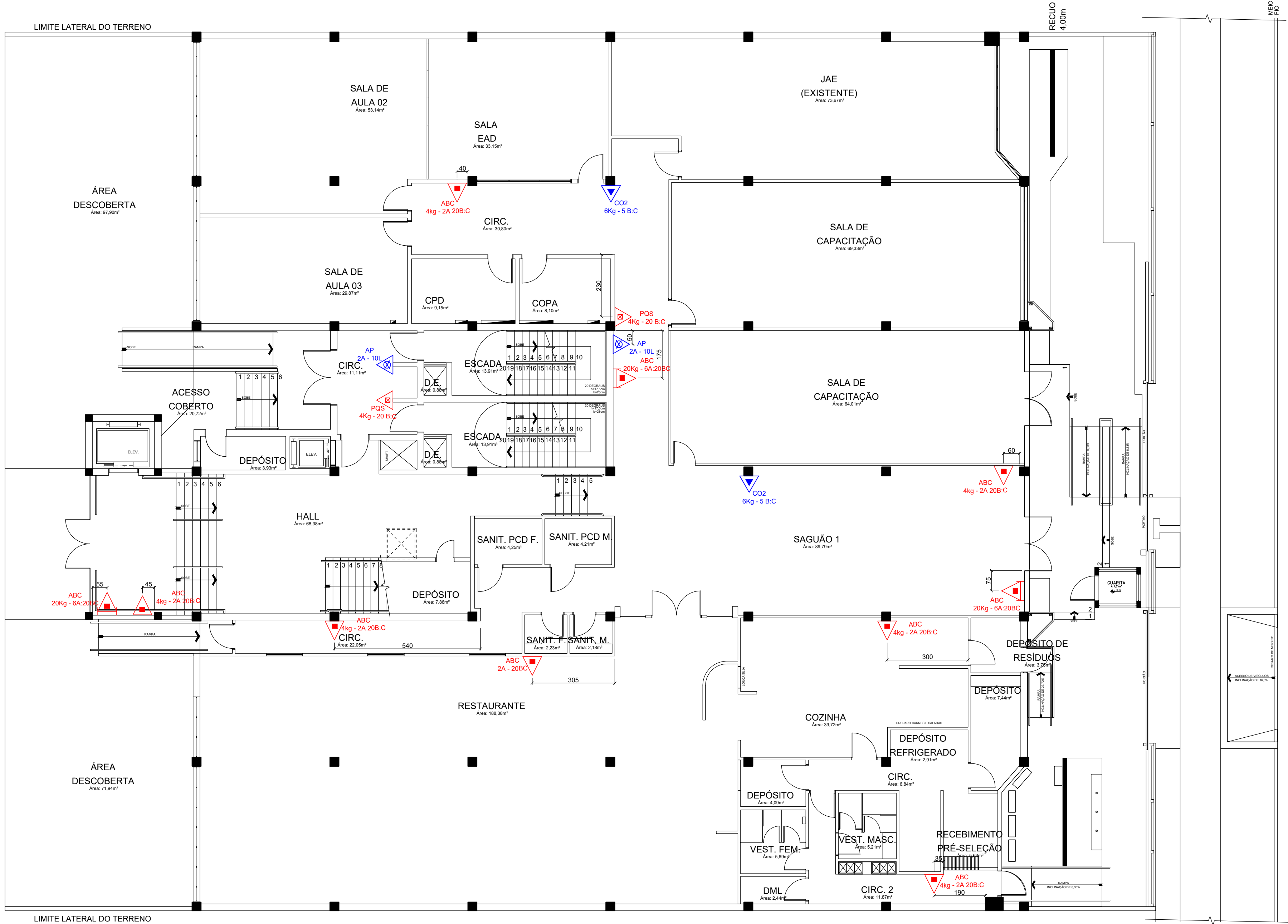
PLANTA BAIXA PAVIMENTO TÉRREO esc.: 1:100
