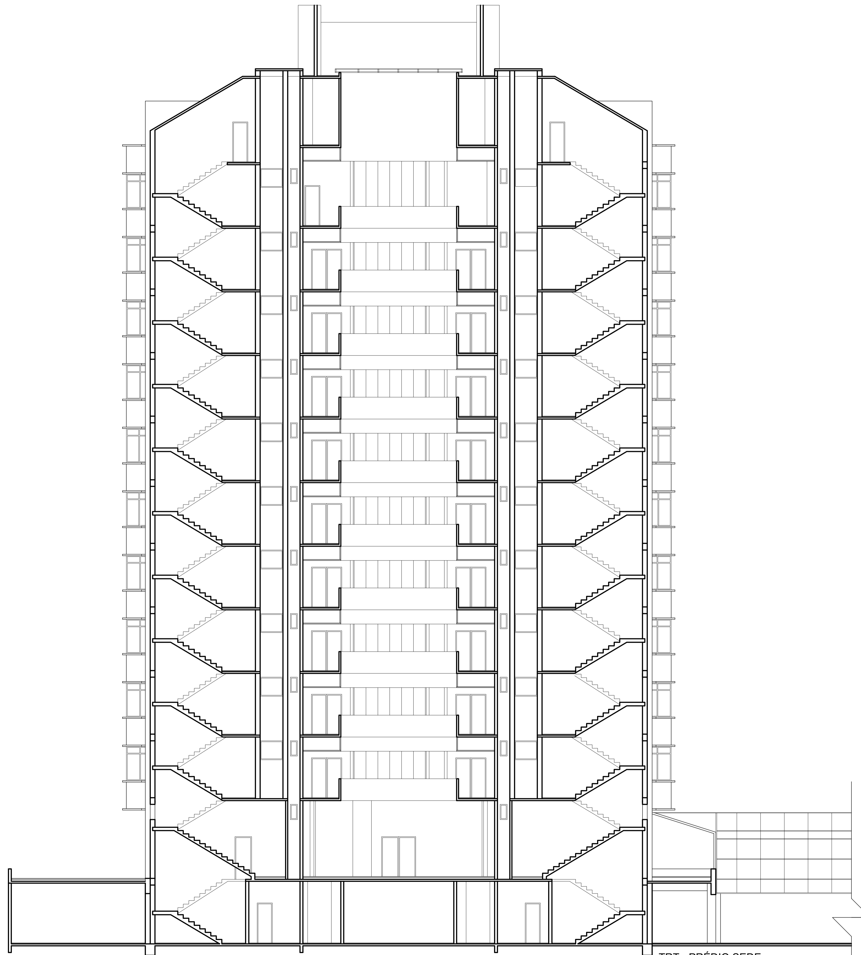
TRT - PRÉDIO SEDE CORTE A-A ESC.: 1/100
