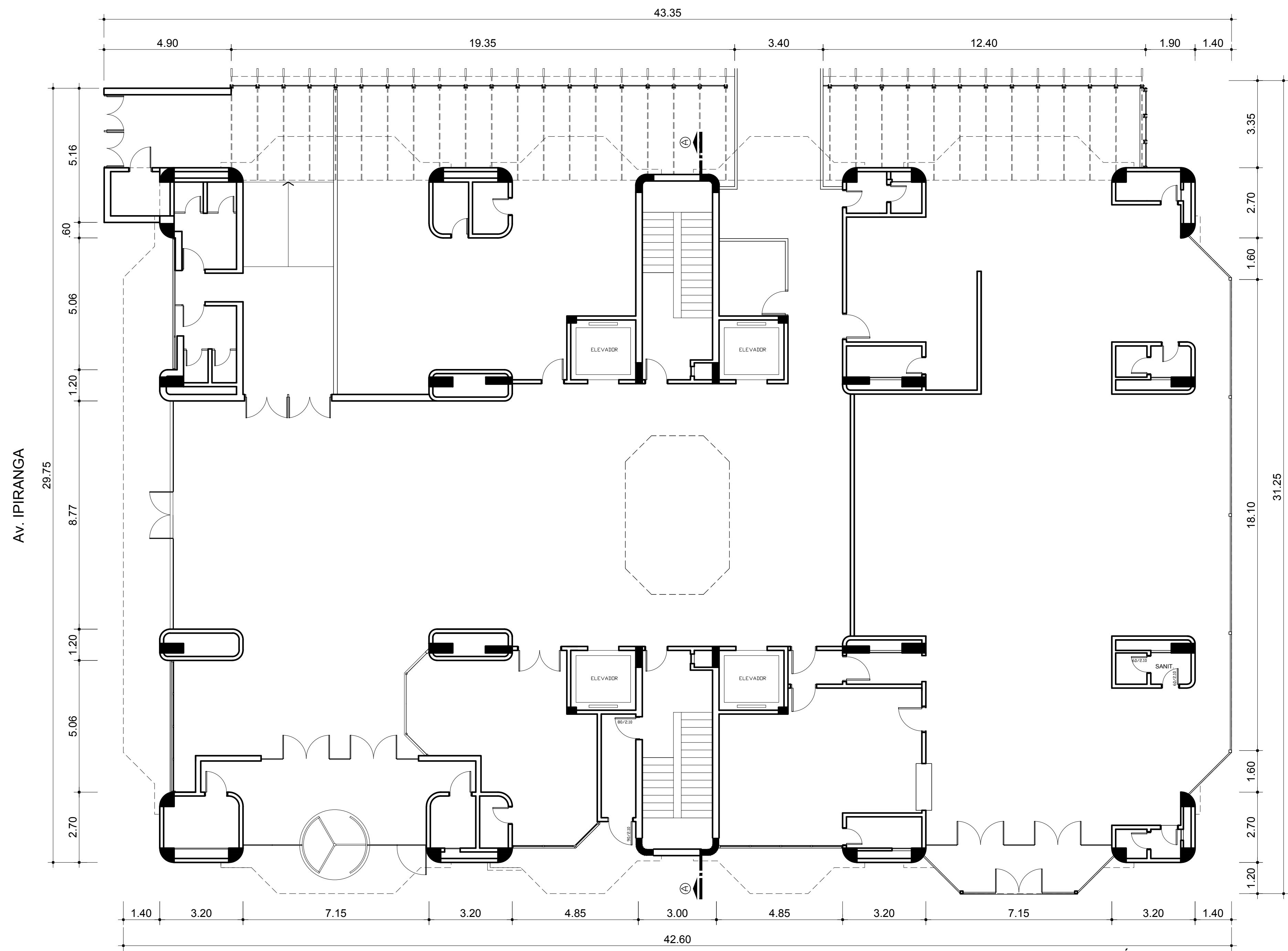
TRT - PRÉDIO SEDE PLANTA BAIXA TÉRREO ESC.: 1/100
