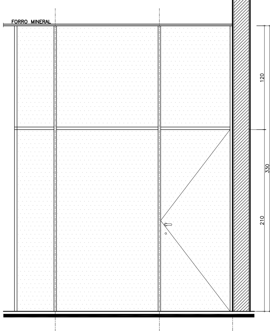
VISTA ESC.: 1/25
