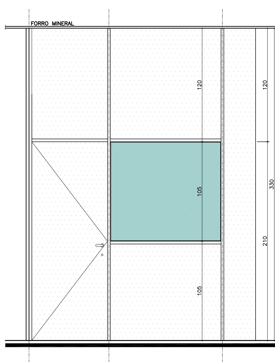
VISTA ESC.: 1/25
