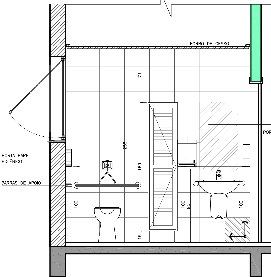
VISTA 05 ESC.: 1/25
