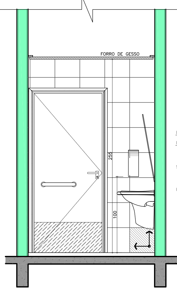
VISTA 02 ESC.: 1/25
