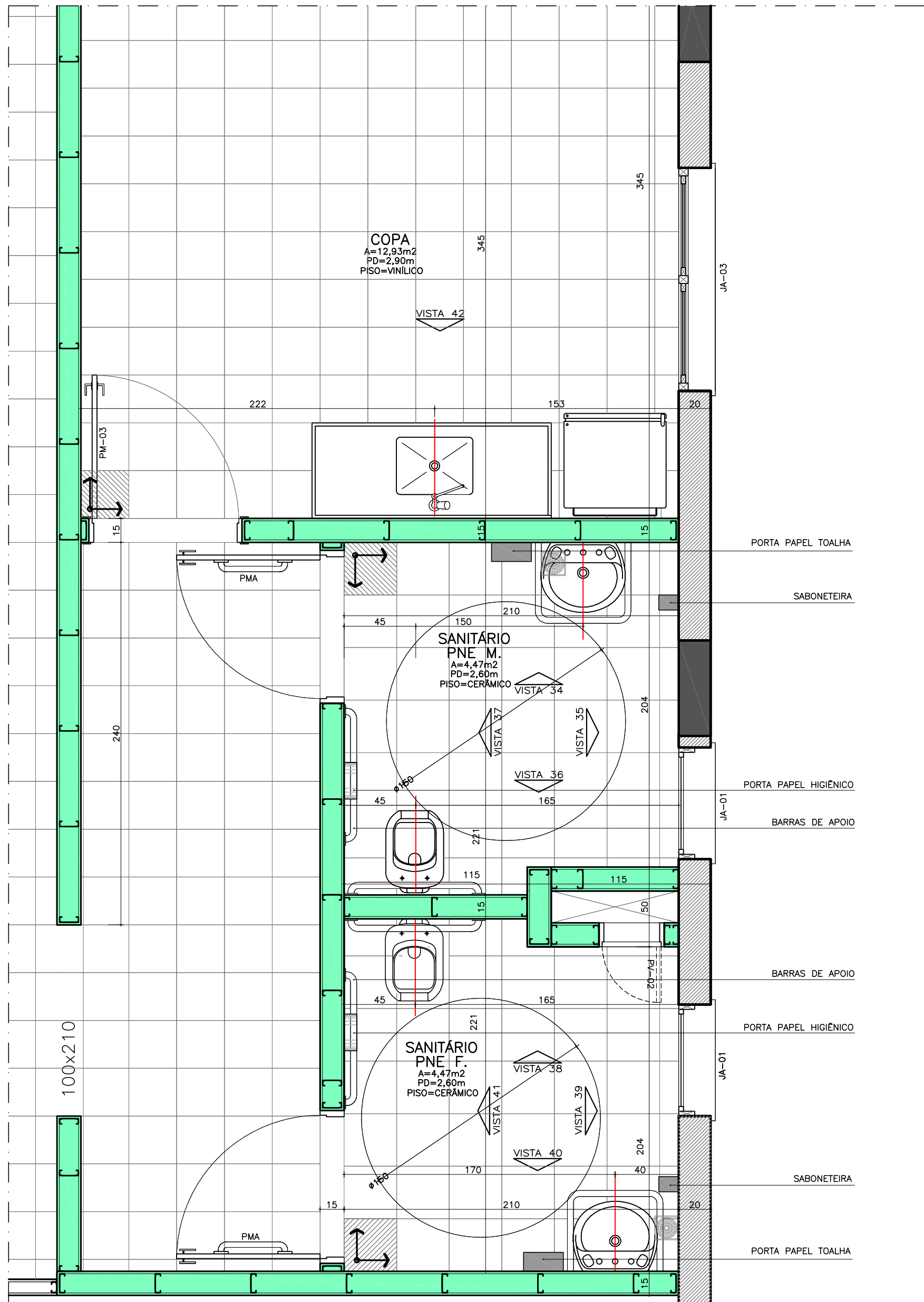
PLANTA BAIXA – SETOR DO 2 AO 6º PAVIMENTO ESC.: 1/50
