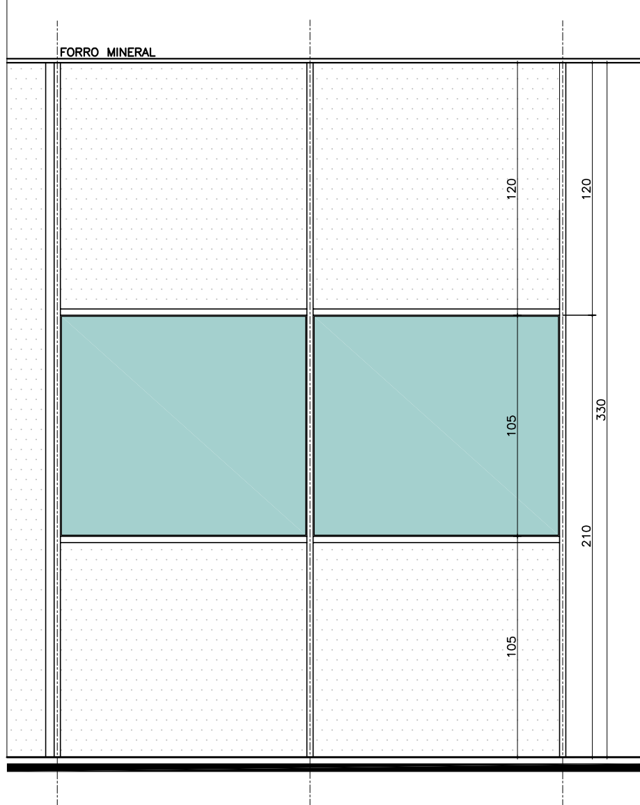
VISTA ESC.: 1/25
