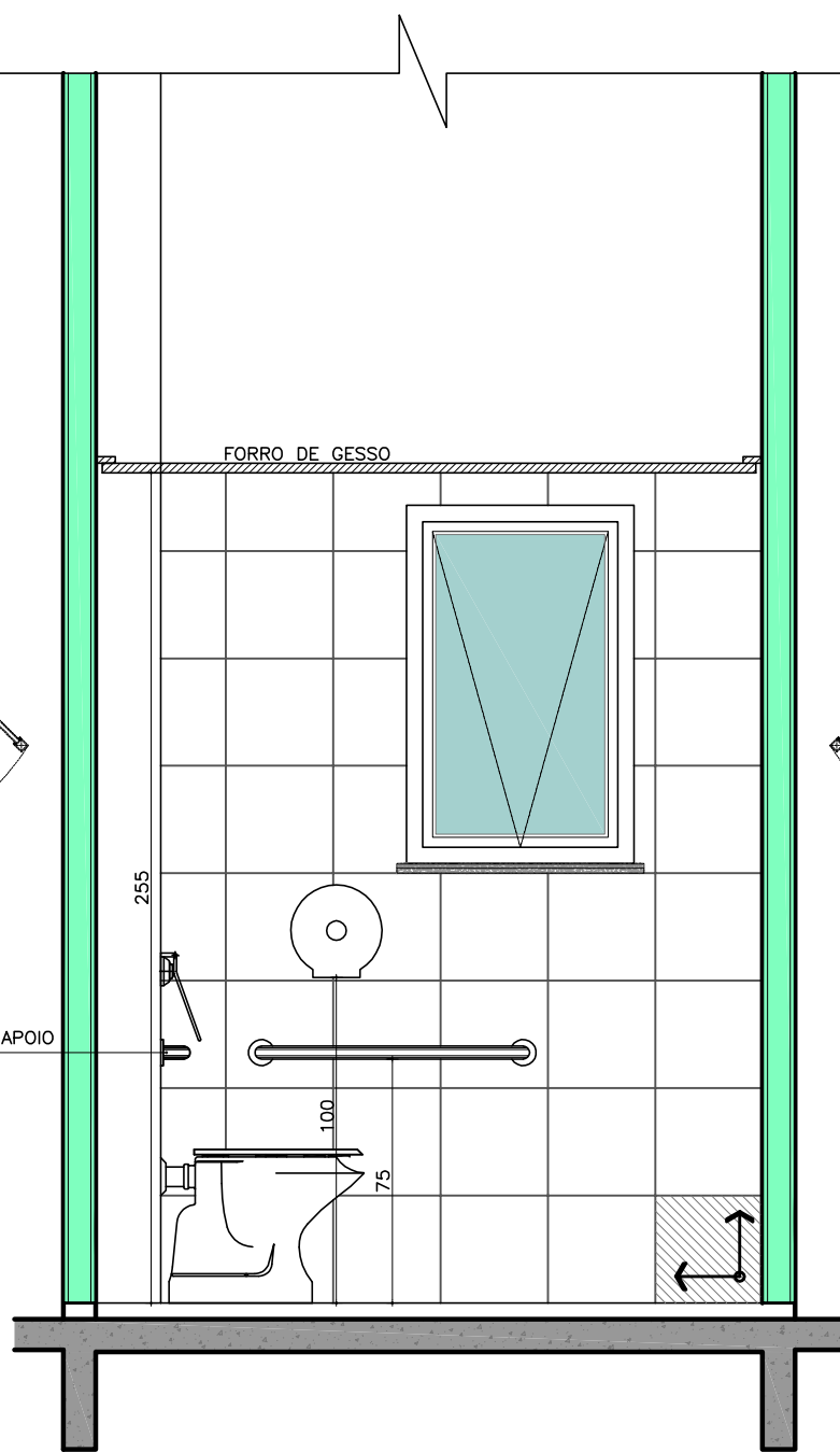
VISTA 22 ESC.: 1/25
