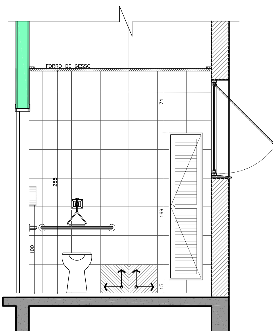
VISTA 38 ESC.: 1/25
