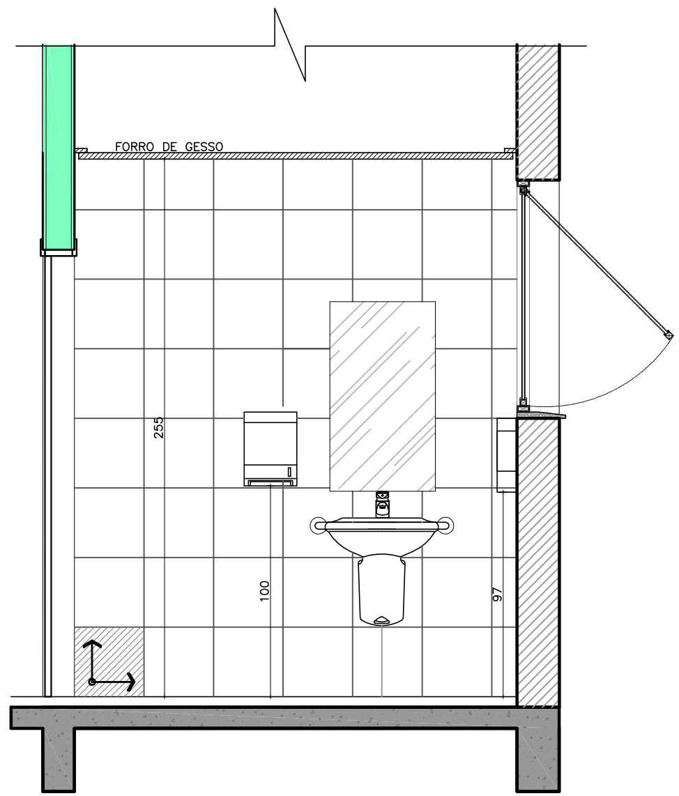
VISTA 34 ESC.: 1/25
