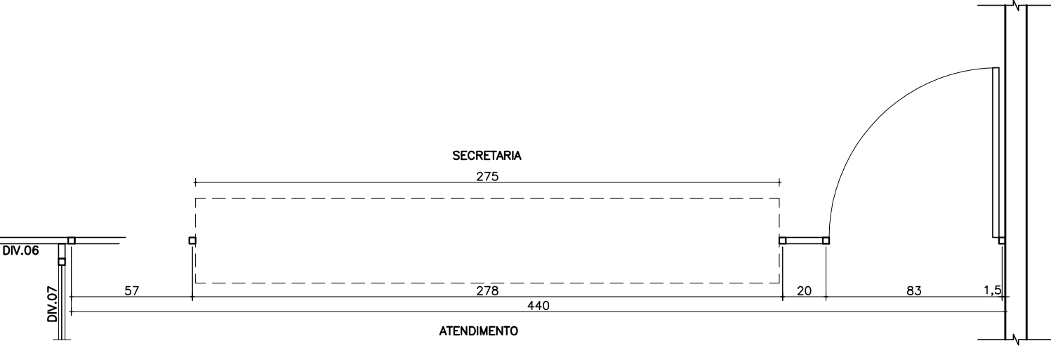
PLANTA BAIXA ESC.: 1/25
