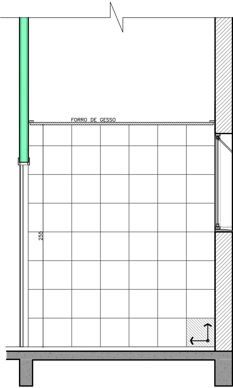
VISTA 17 ESC.: 1/25
