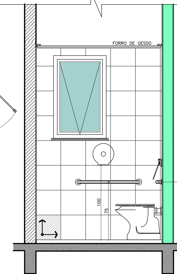
VISTA 08 ESC.: 1/25
