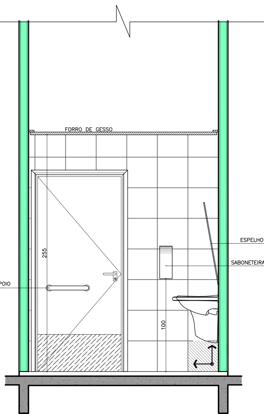
VISTA 24 ESC.: 1/25
