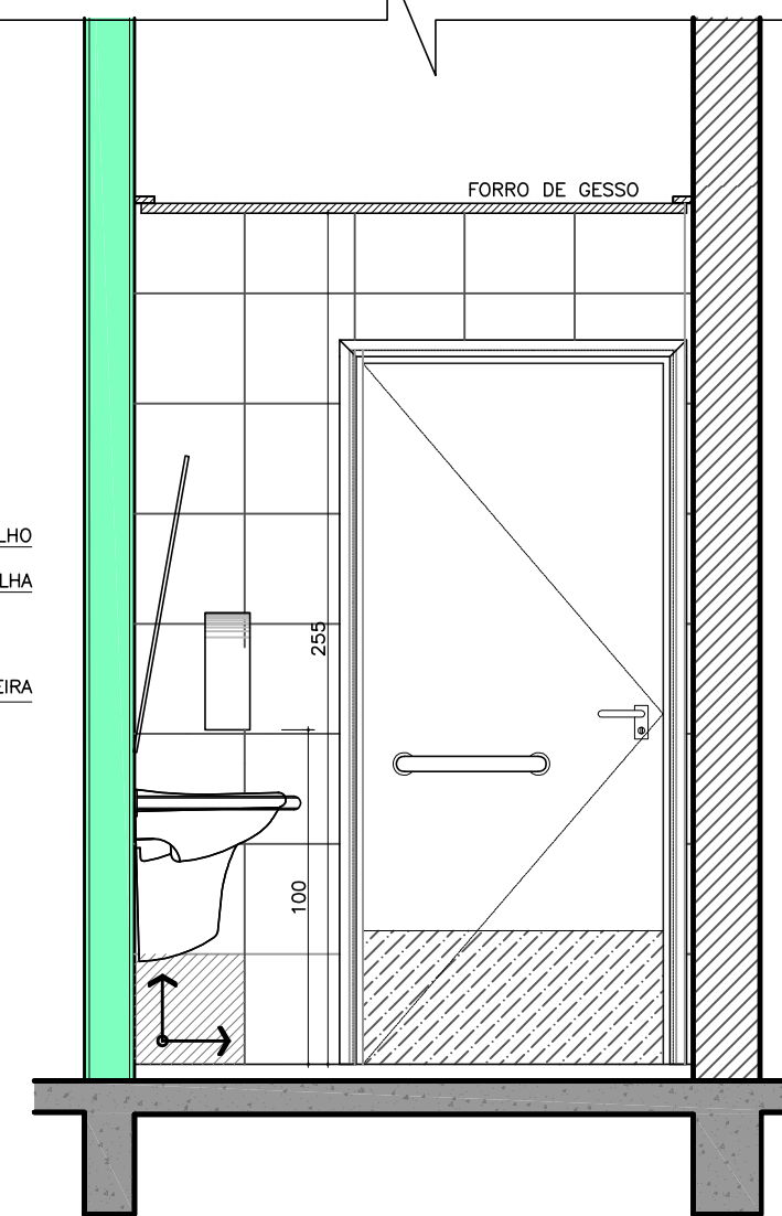
VISTA 06 ESC.: 1/25
