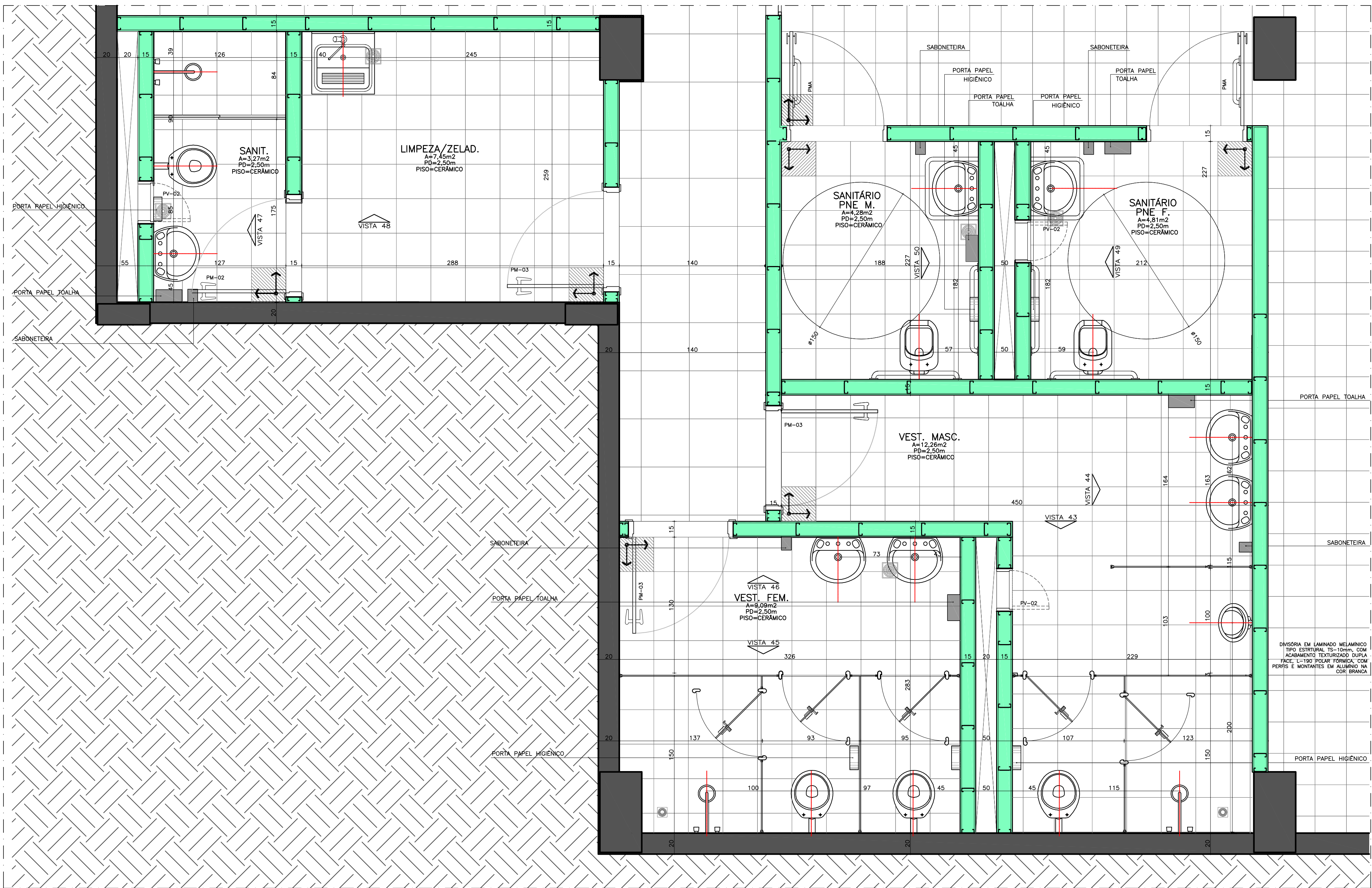
PLANTA BAIXA – SETOR SUBSOLO 01
