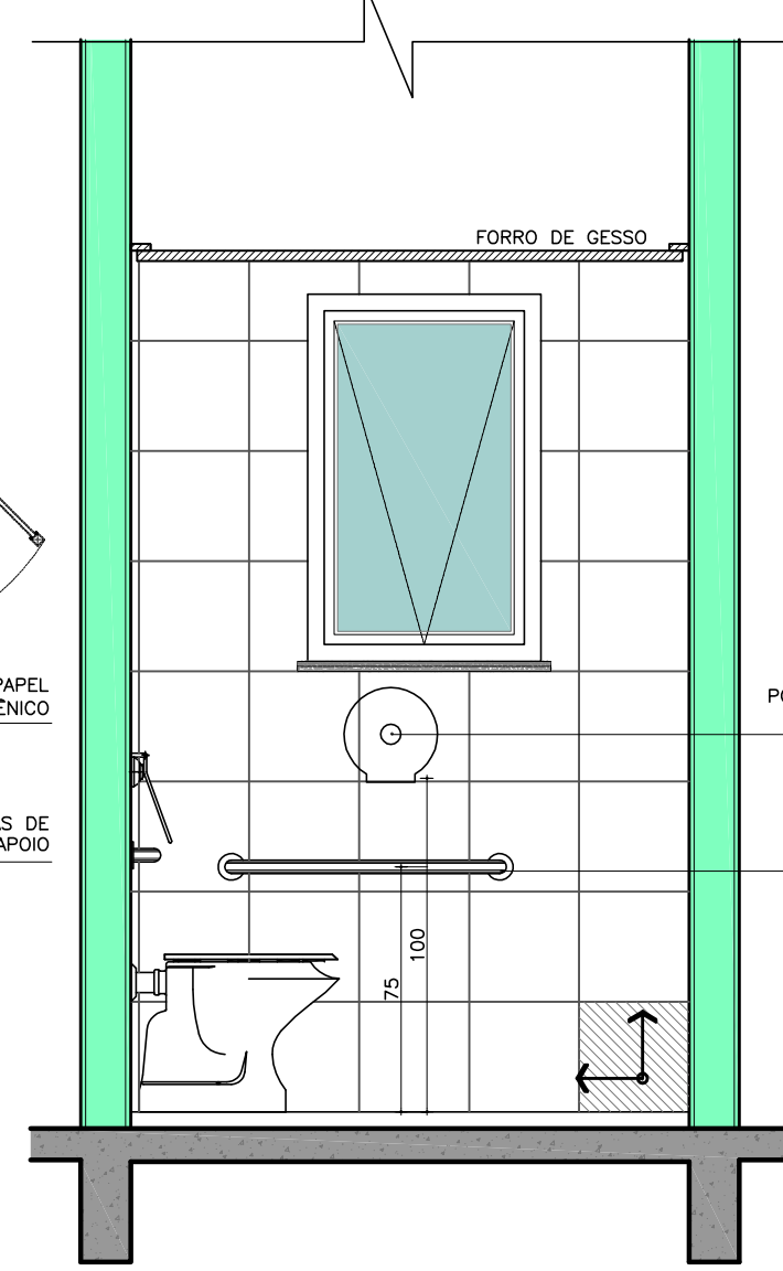
VISTA 04 ESC.: 1/25
