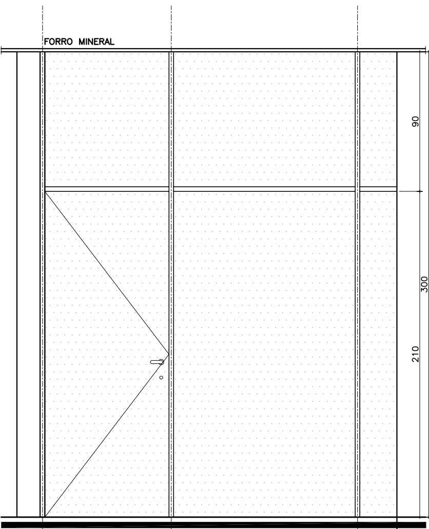
VISTA ESC.: 1/25
