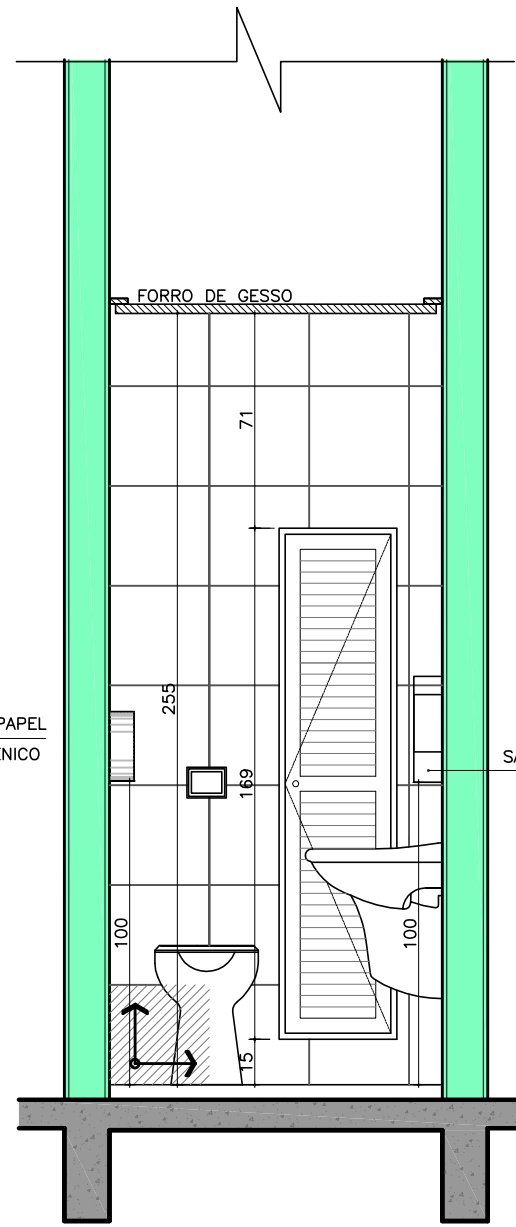
VISTA 10 ESC.: 1/25
