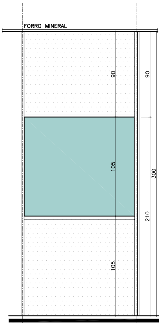
VISTA ESC.: 1/25
