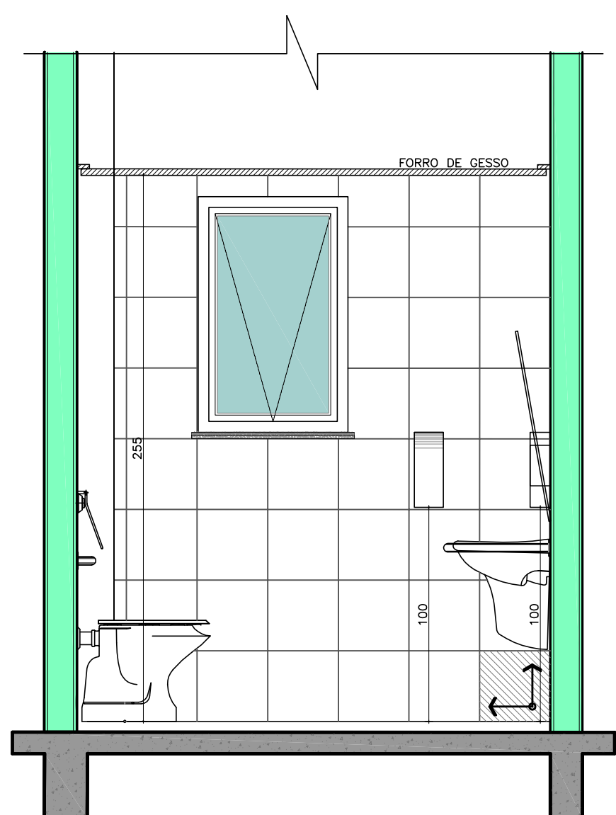
VISTA 39 ESC.: 1/25
