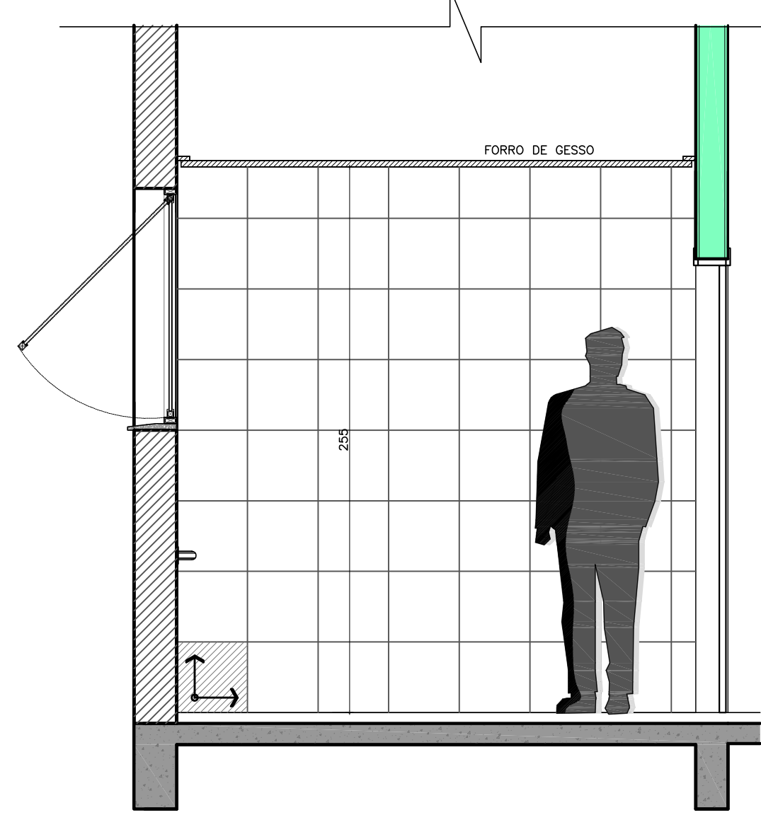
VISTA 01 ESC.: 1/25
