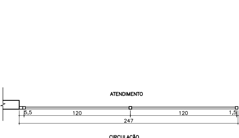
PLANTA BAIXA ESC.: 1/25
