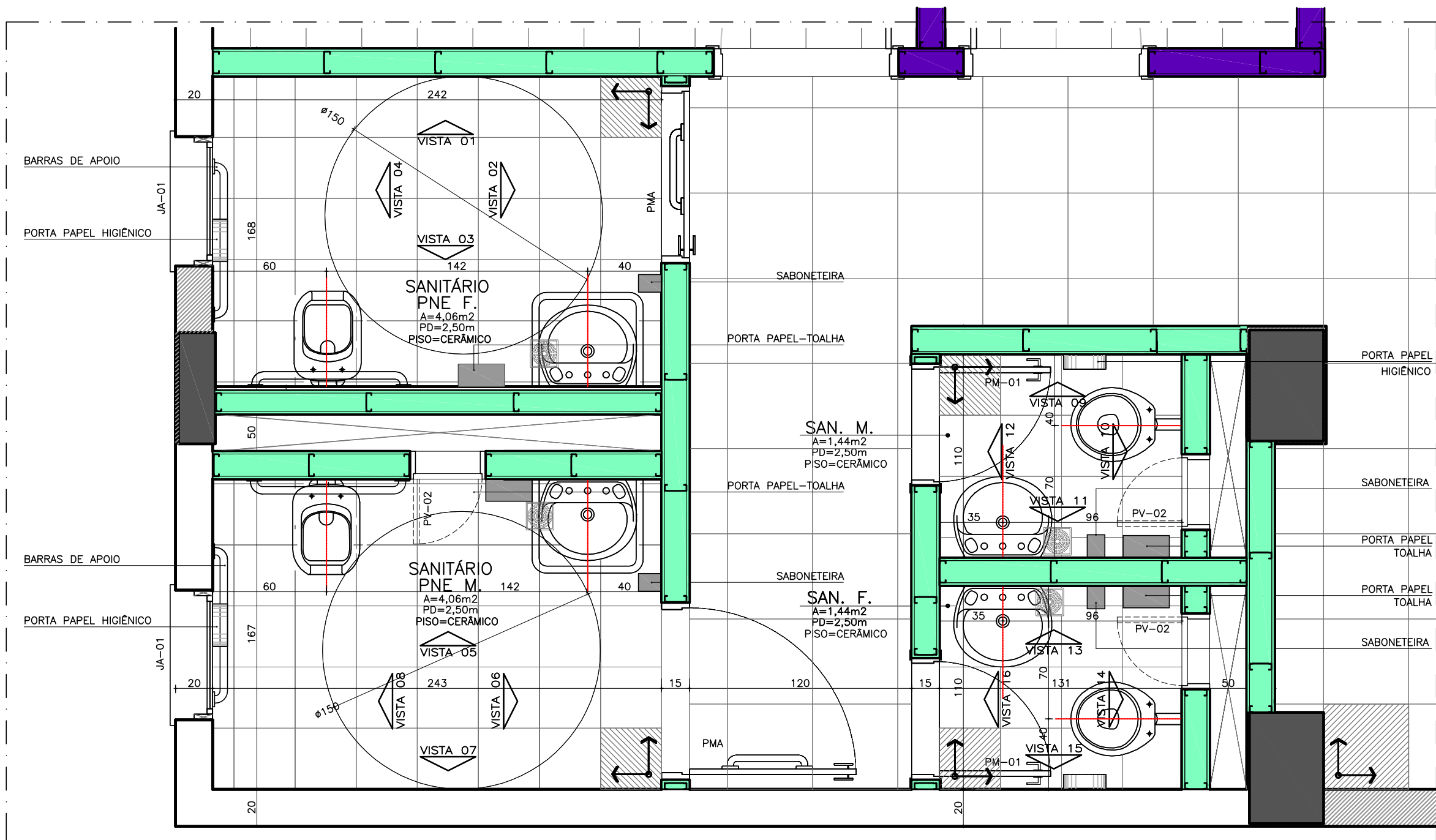
PLANTA BAIXA – SETOR TÉRREO E DO 2 AO 6º PAVIMENTO ESC.: 1/50
