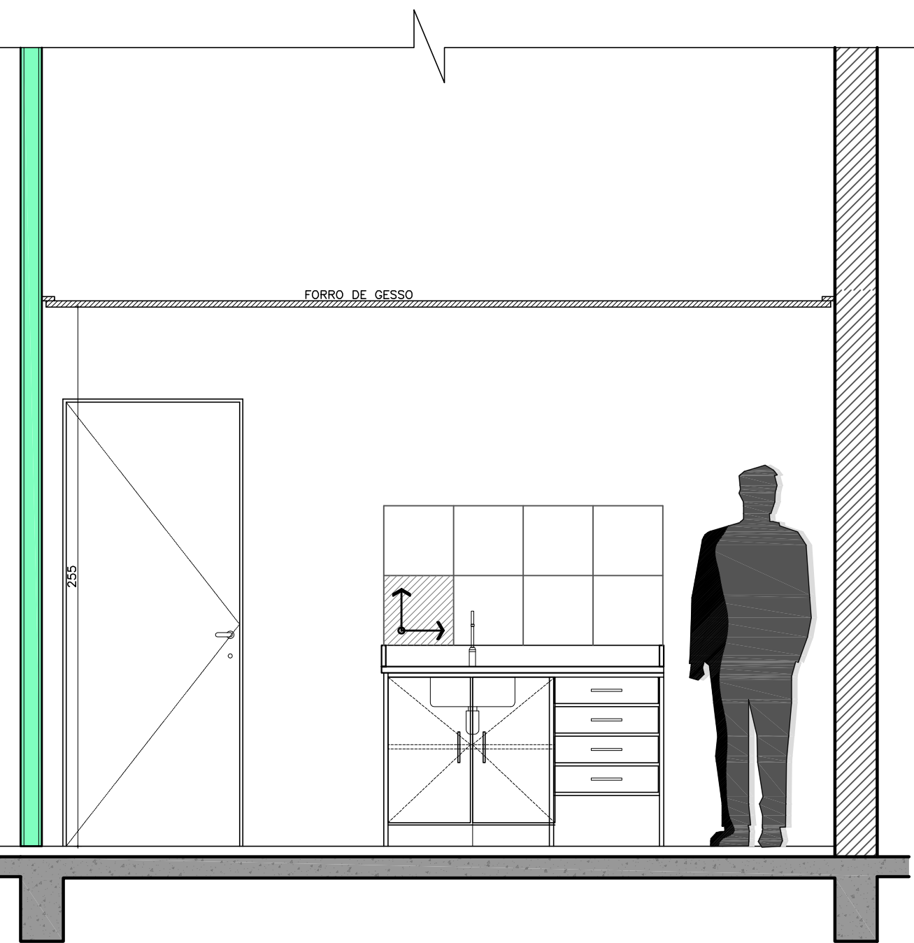
VISTA 25 ESC.: 1/25
