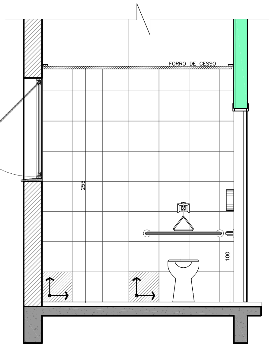
VISTA 36 ESC.: 1/25
