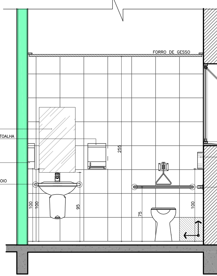
VISTA 03 ESC.: 1/25
