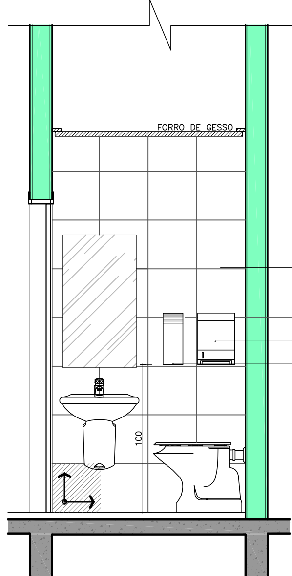
VISTA 13 ESC.: 1/25
