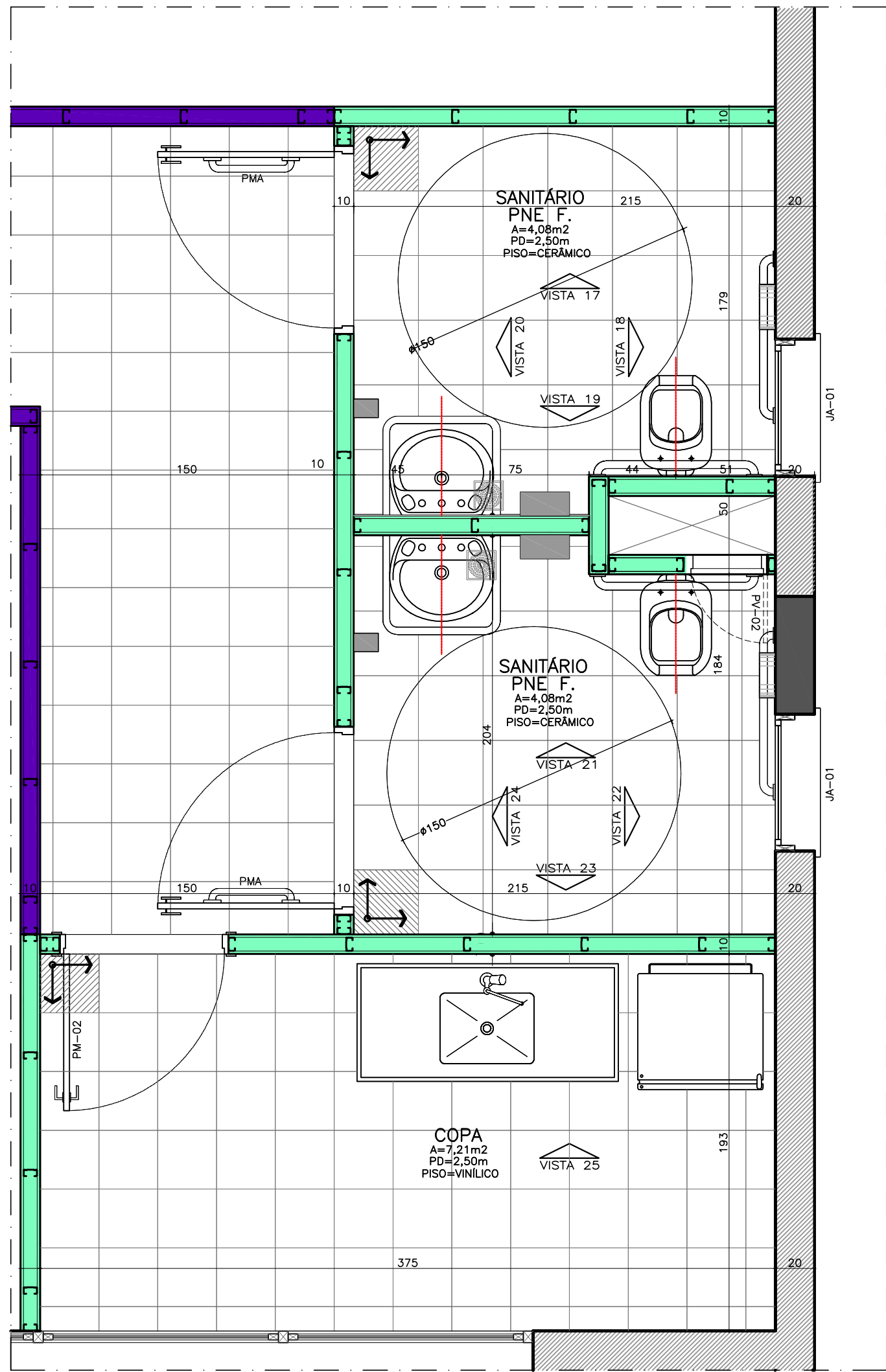
PLANTA BAIXA – SETOR TÉRREO ESC.: 1/50
