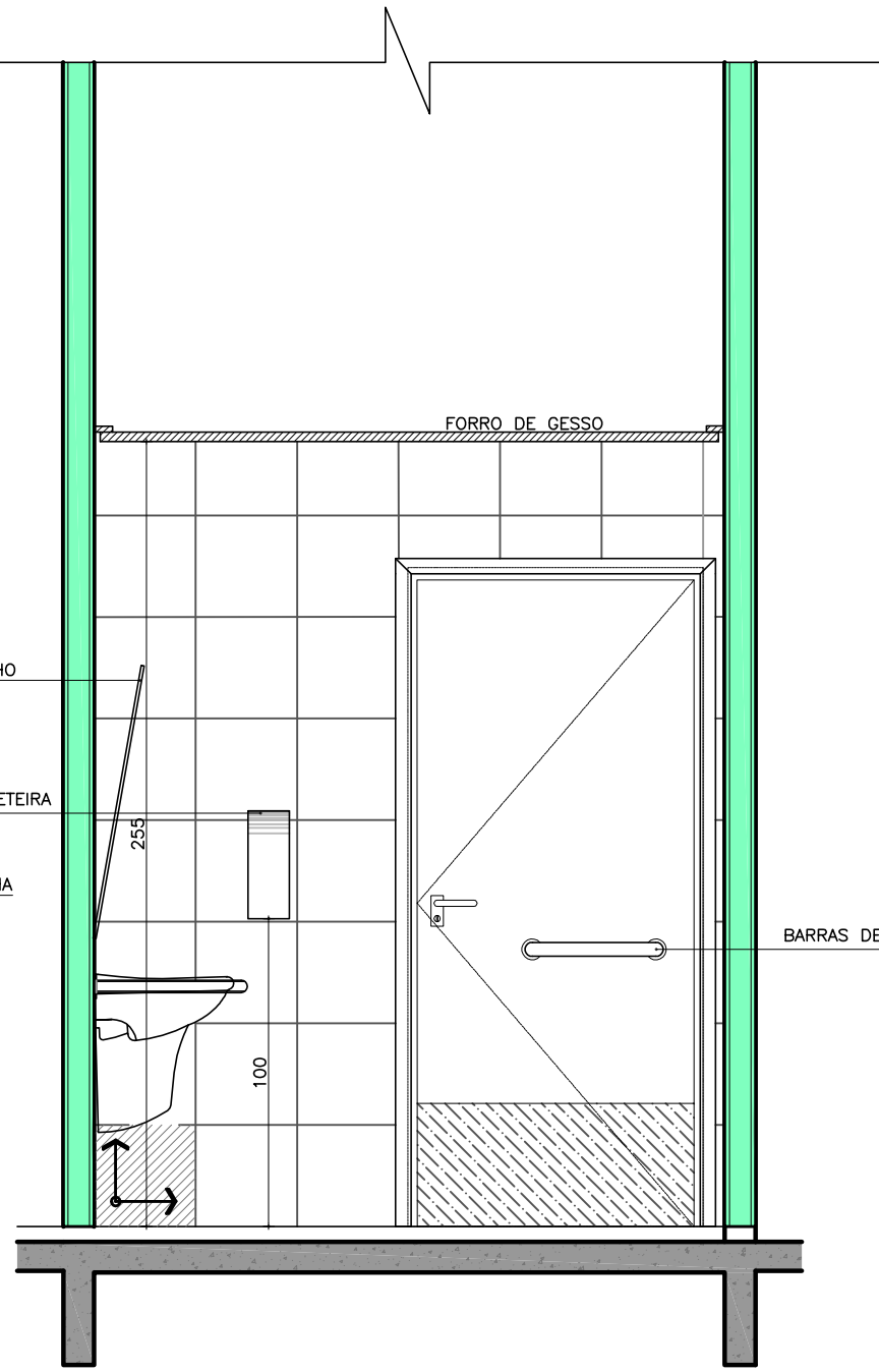
VISTA 20 ESC.: 1/25
