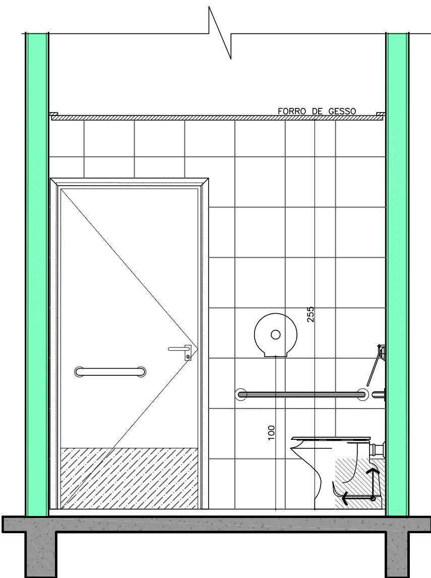
VISTA 41 ESC.: 1/25
