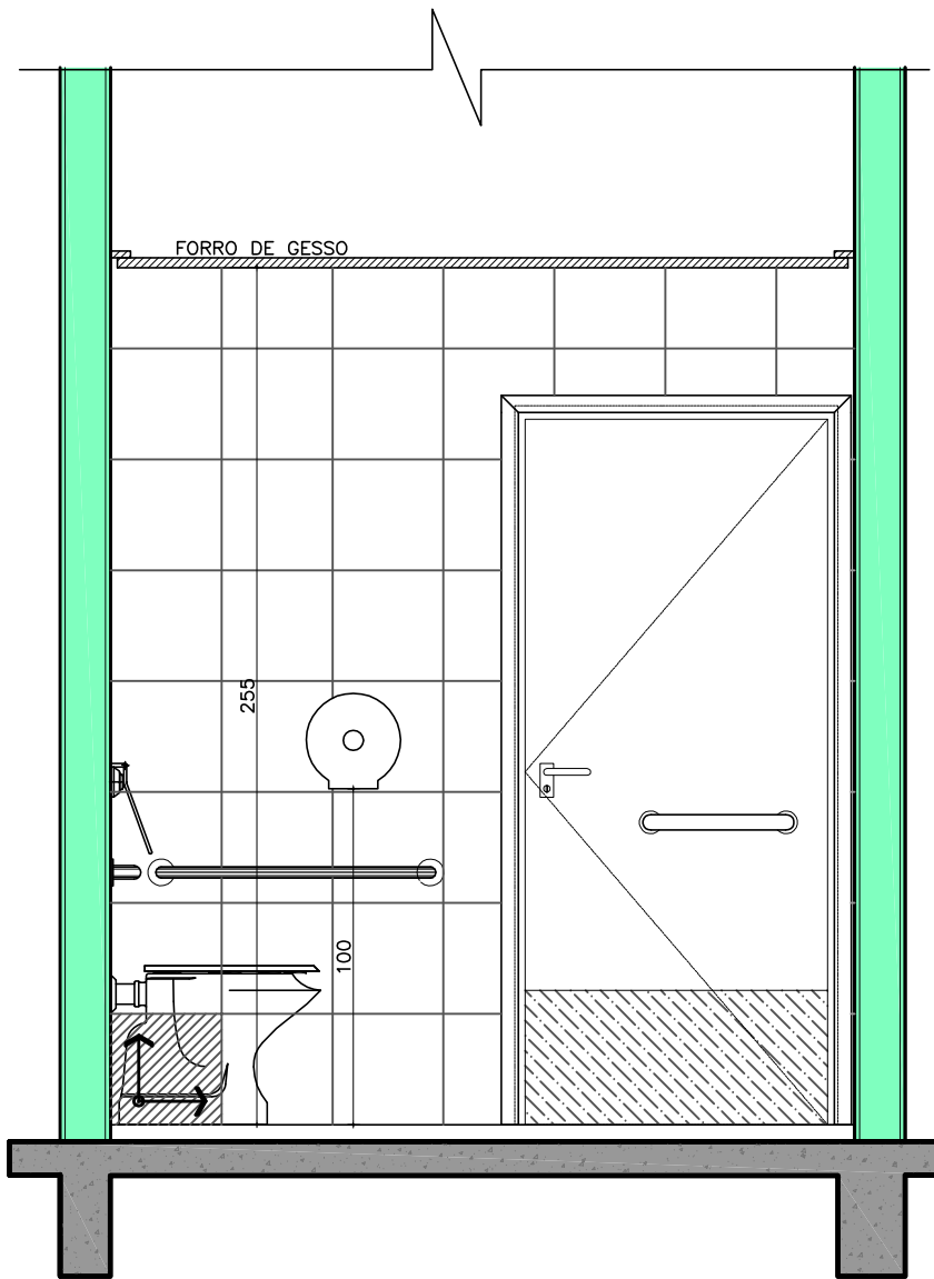
VISTA 37 ESC.: 1/25
