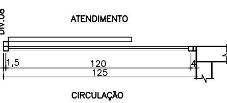
PLANTA BAIXA ESC.: 1/25
