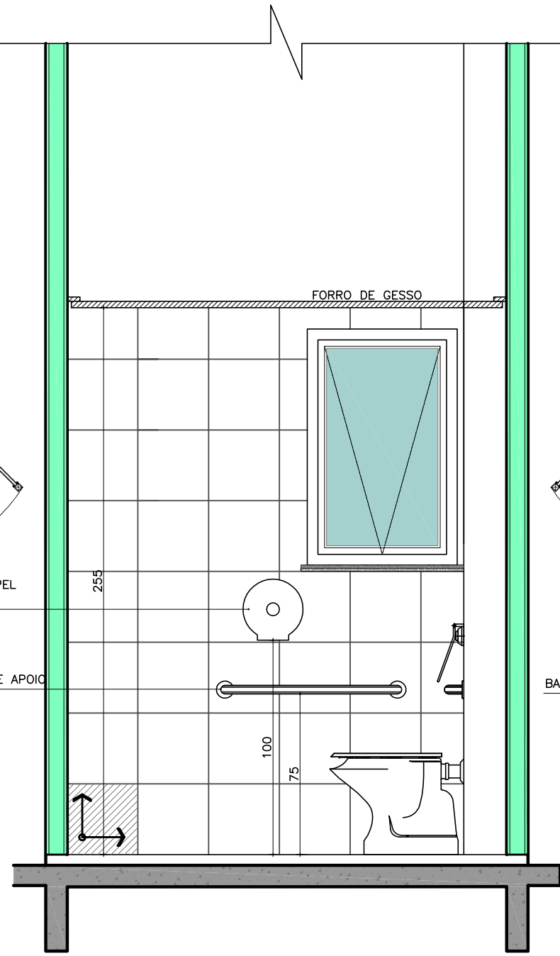
VISTA 18 ESC.: 1/25
