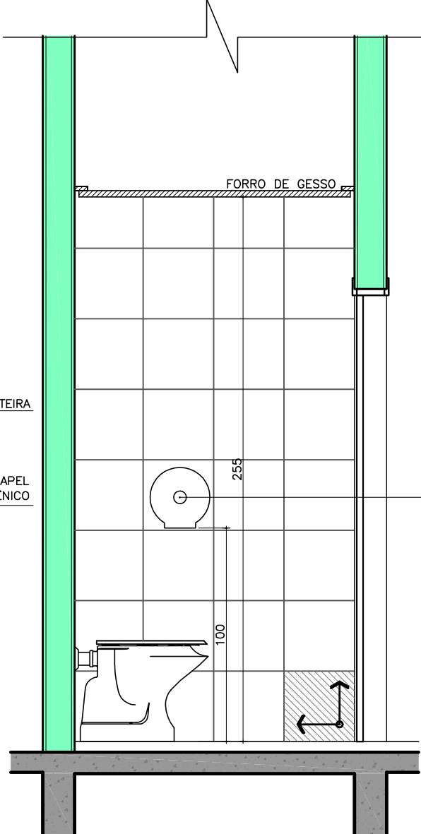
VISTA 15 ESC.: 1/25
