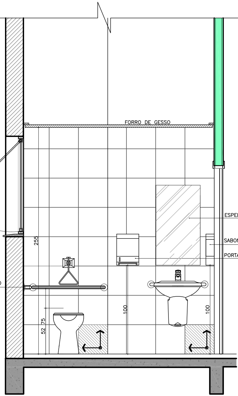
VISTA 19 ESC.: 1/25
