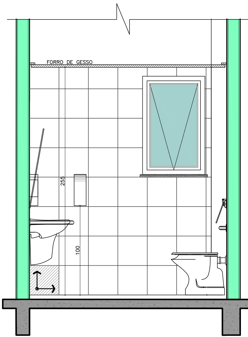
VISTA 35 ESC.: 1/25
