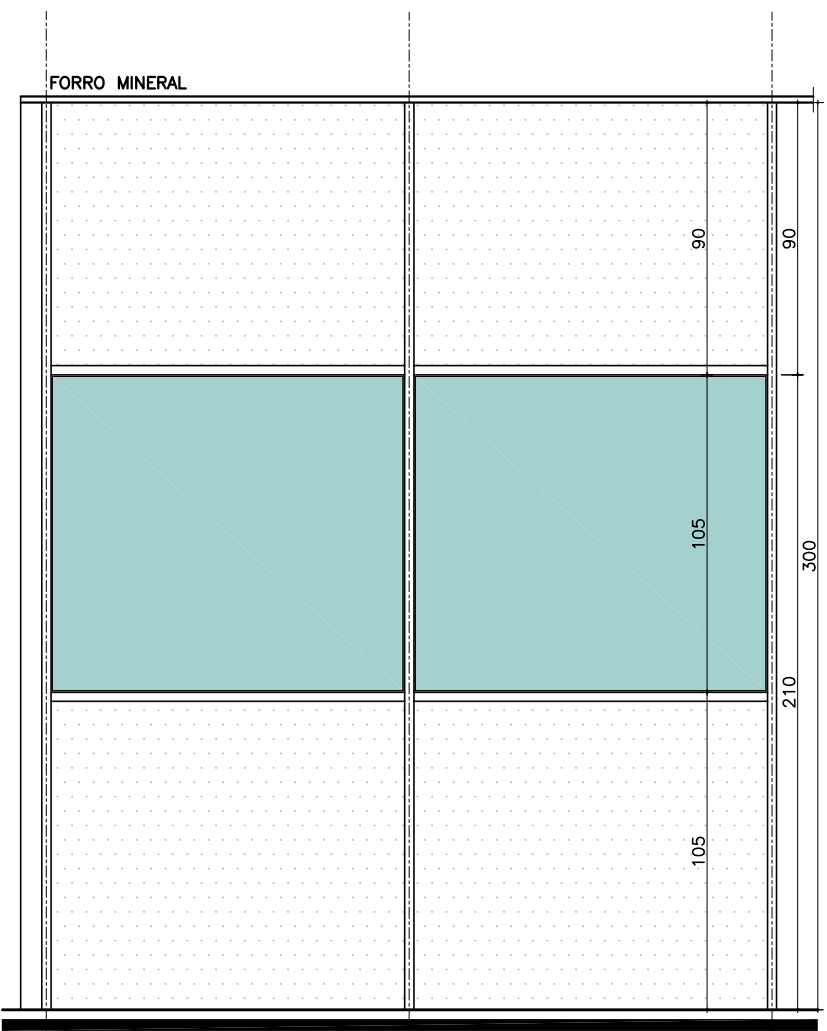
VISTA ESC.: 1/25
