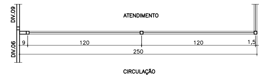
PLANTA BAIXA ESC.: 1/25
