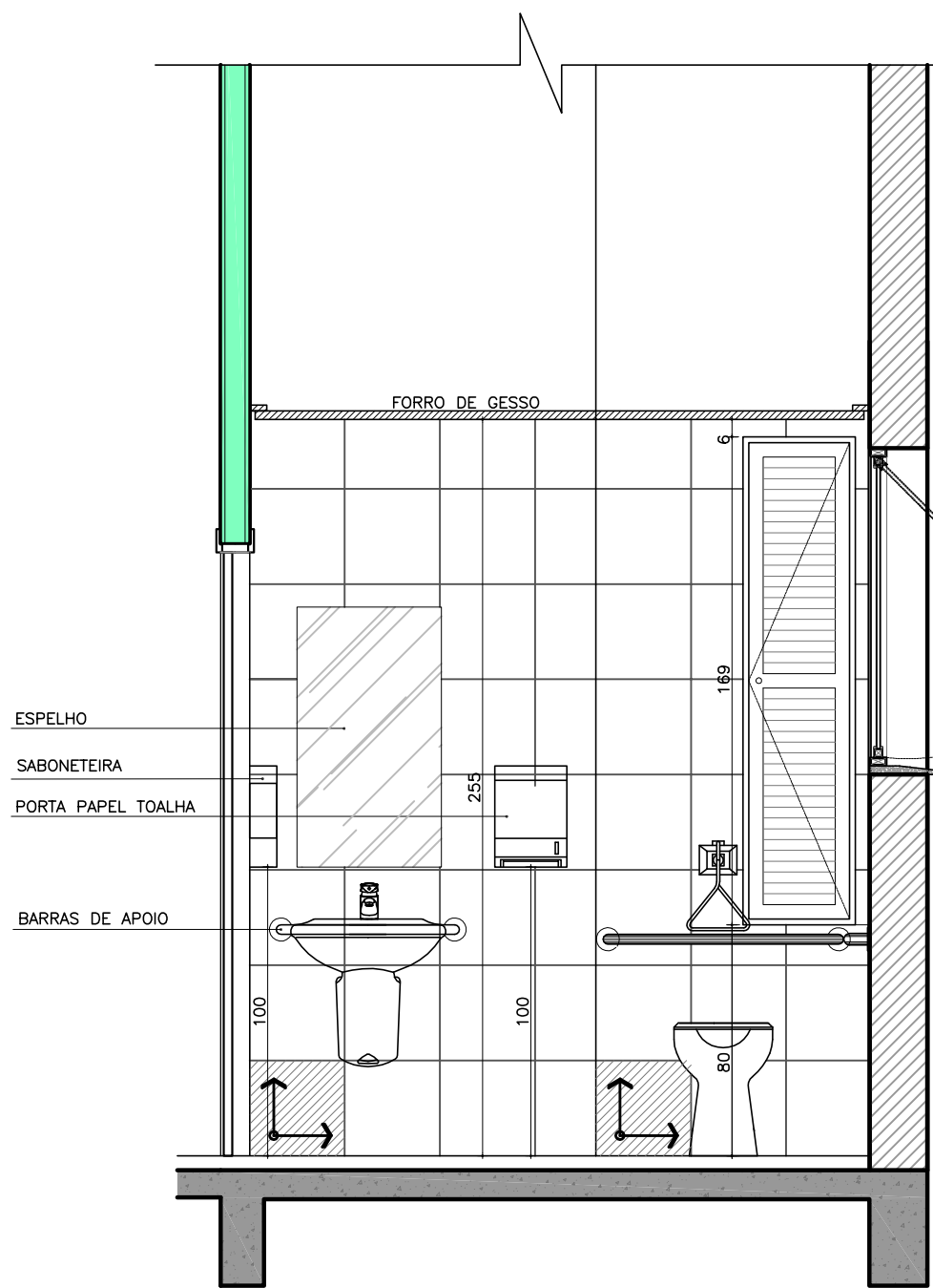
VISTA 21 ESC.: 1/25
