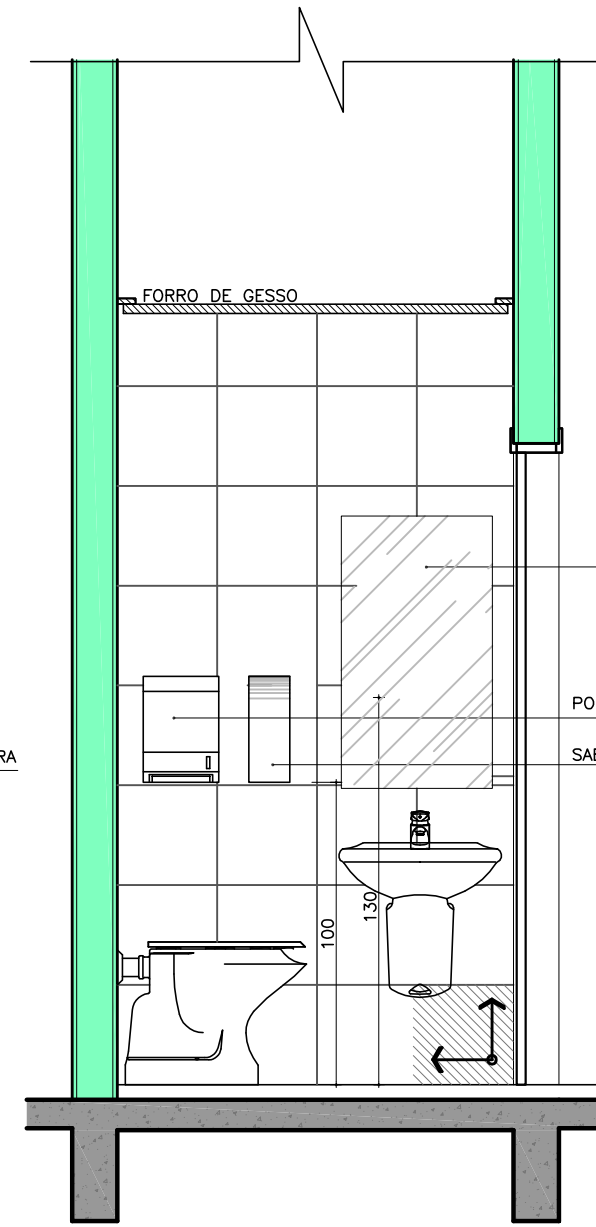
VISTA 11 ESC.: 1/25
