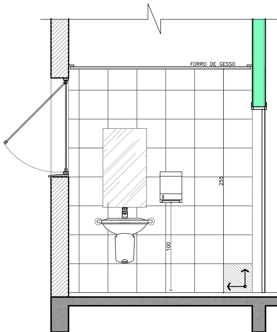
VISTA 40 ESC.: 1/25
