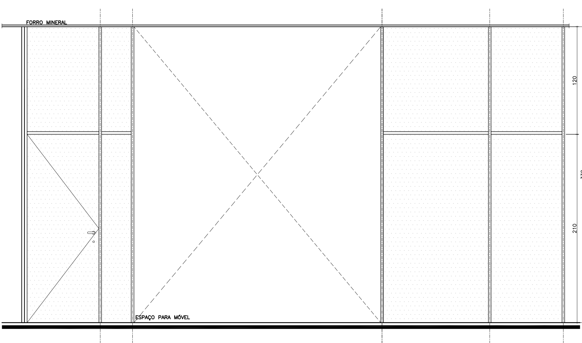
VISTA ESC.: 1/25
