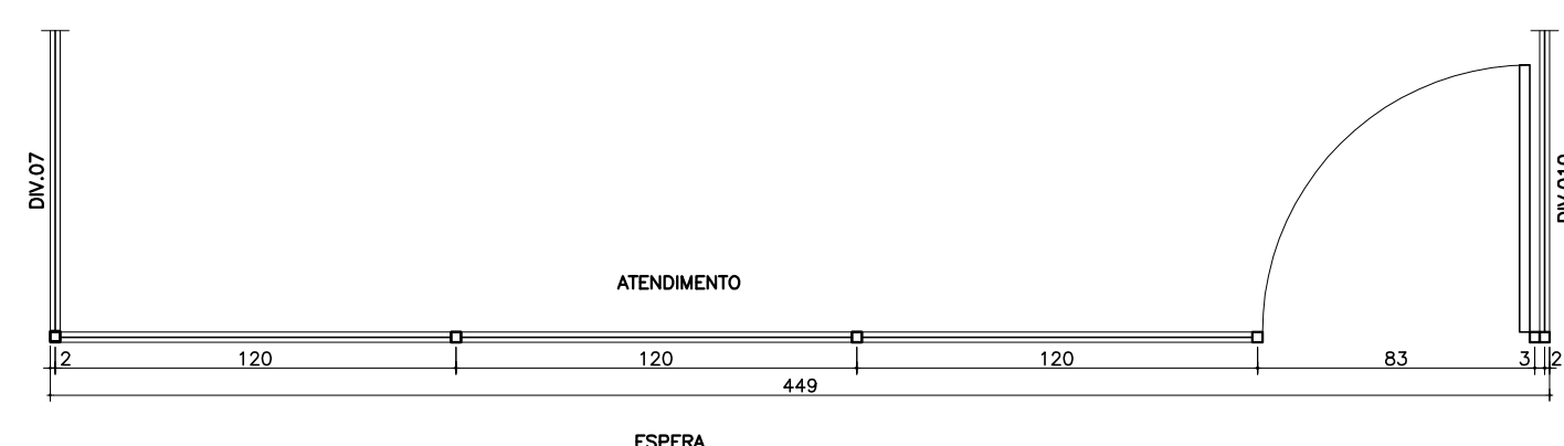
PLANTA BAIXA ESC.: 1/25
