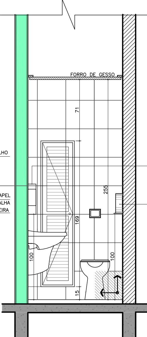
VISTA 14 ESC.: 1/25
