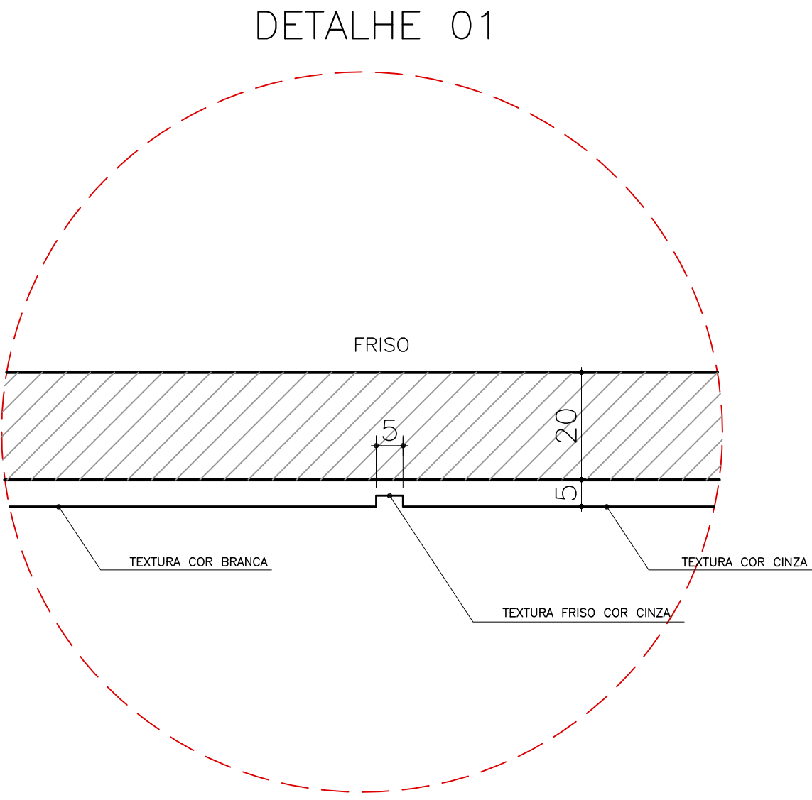
DETALHE 01 ESC.: 1/10
