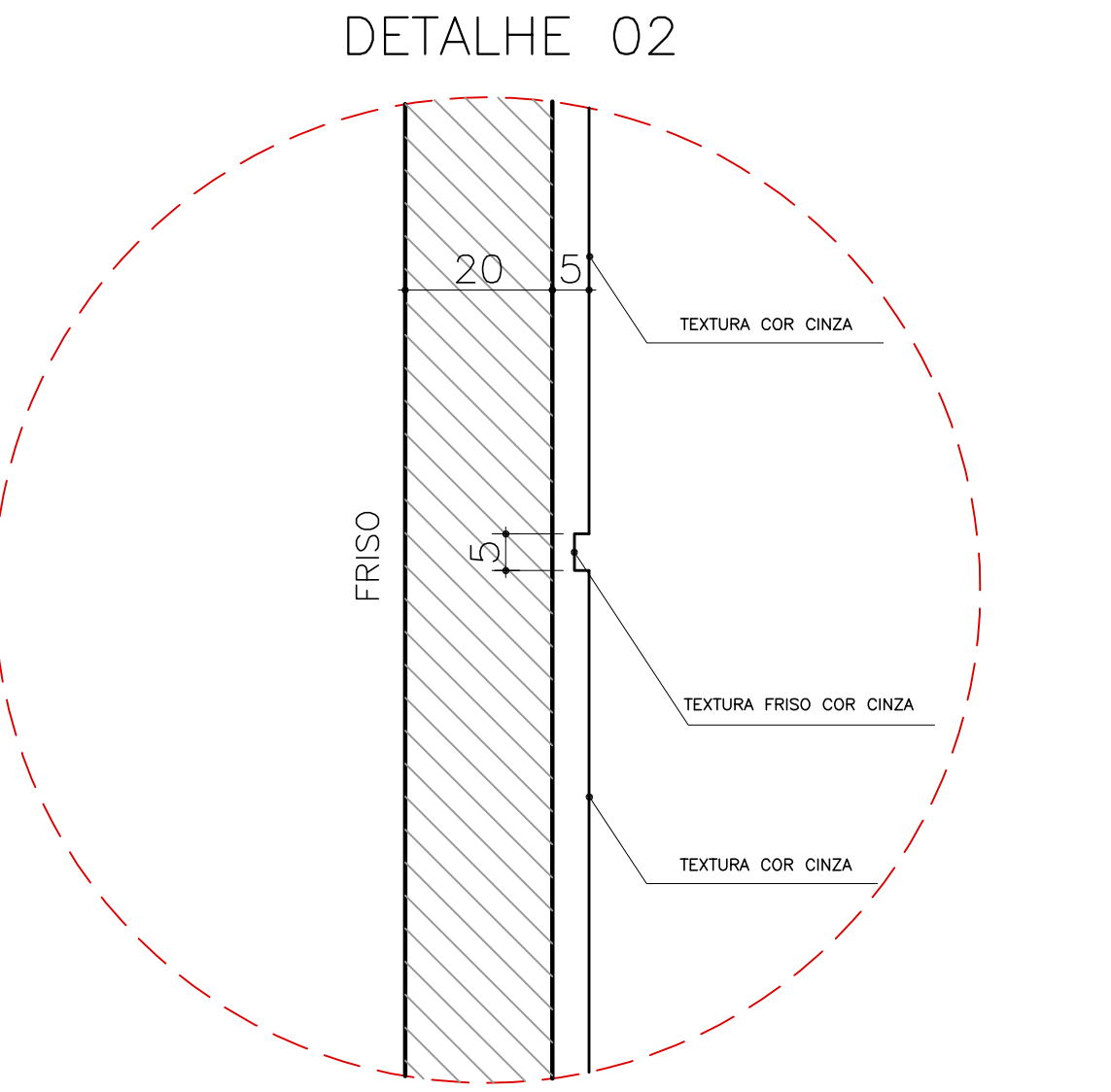
DETALHE 02 ESC.: 1/10
