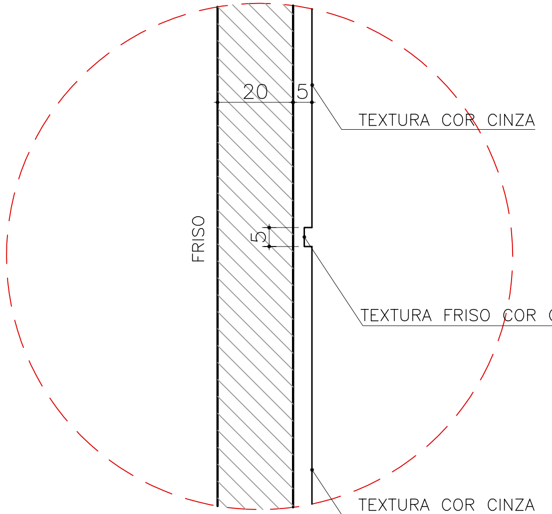
DETALHE 02
