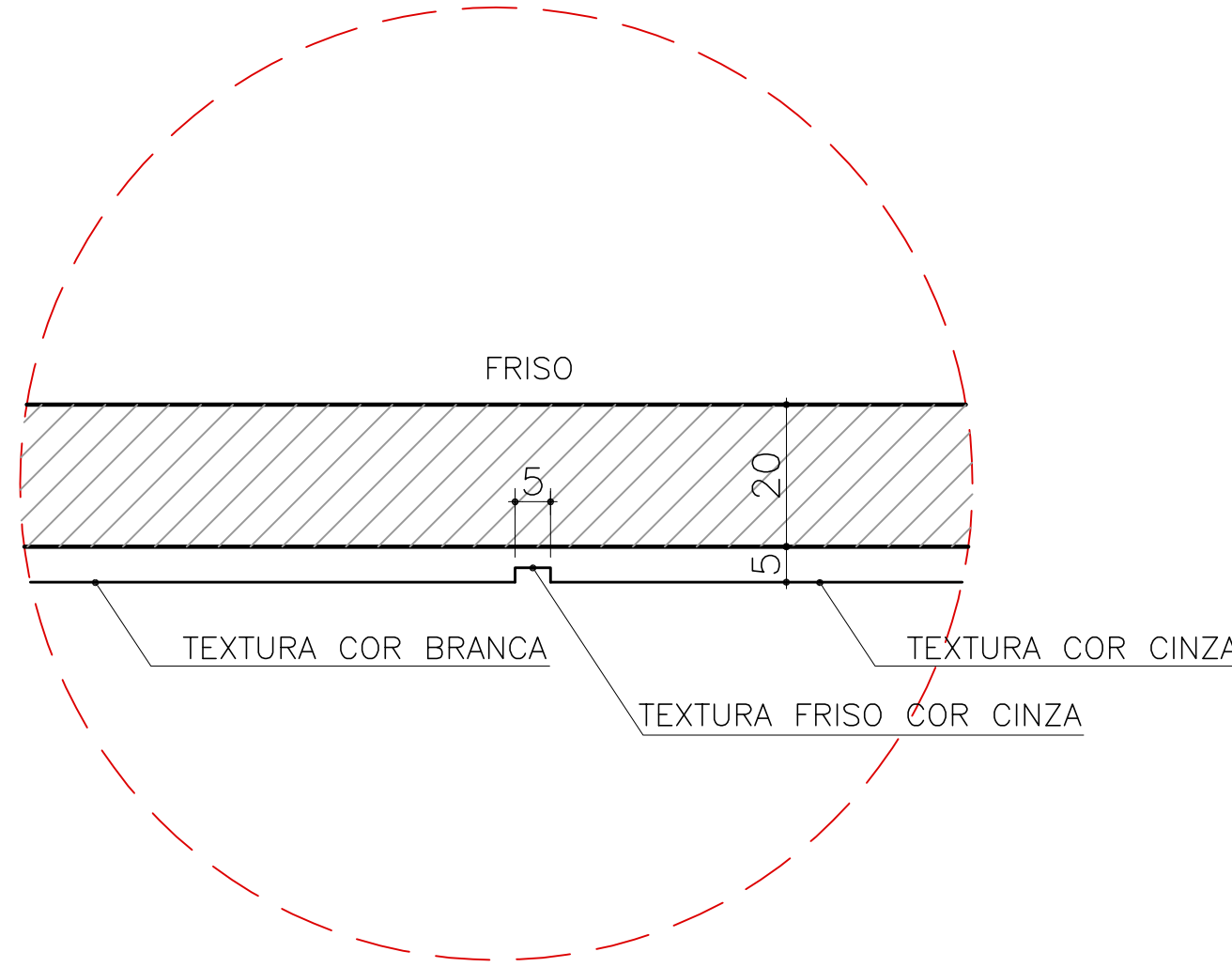
DETALHE 01
