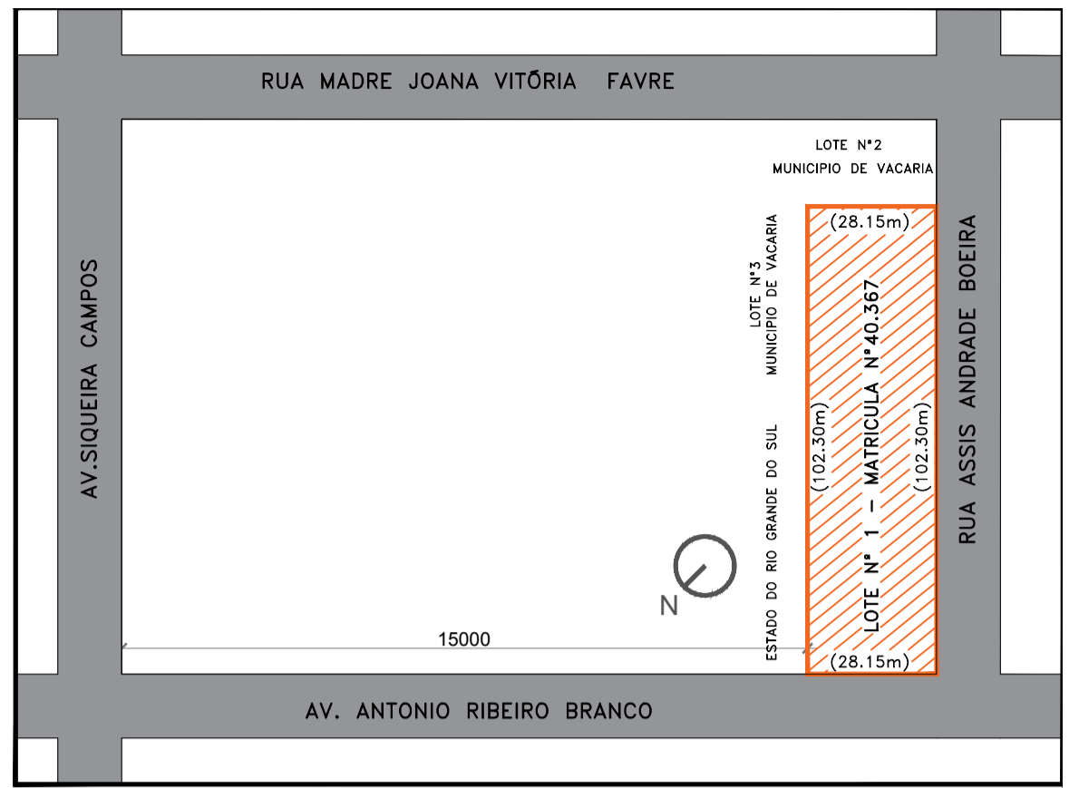
SITUAÇÃO ESCALA= 1/1500
