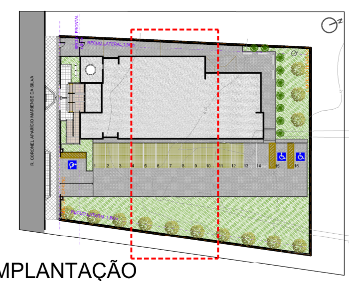
IMPLANTAÇÃO ESCALA= 1/750
