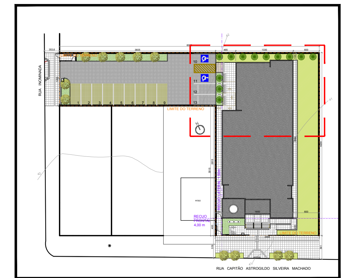
IMPLANTAÇÃO ESCALA= 1:500
